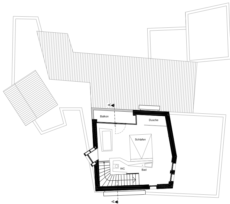
Grundriss 2. Obergeschoss
