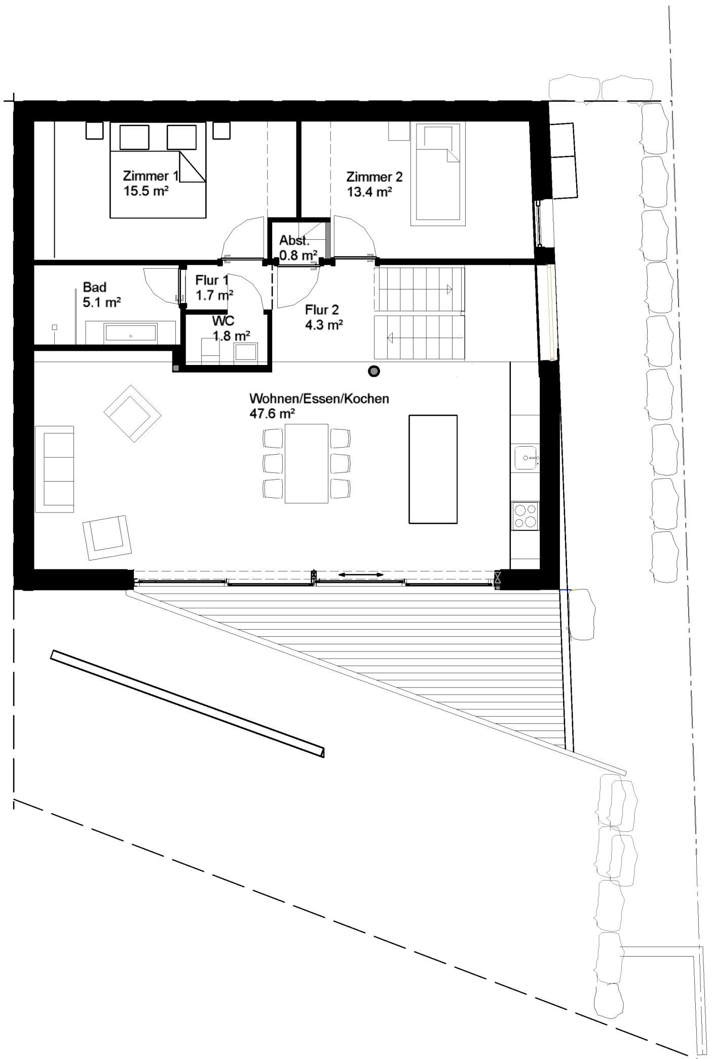
Grundriss OG
