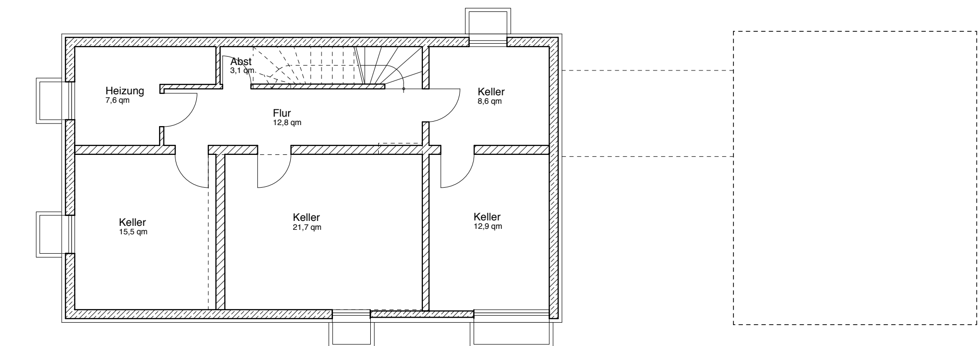
Grundriss Kellergeschoss
