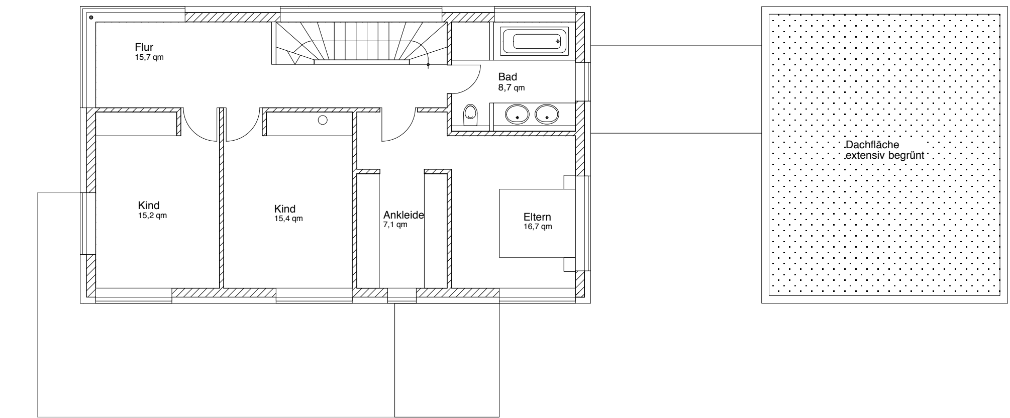
Grundriss 1. Obergeschoss
