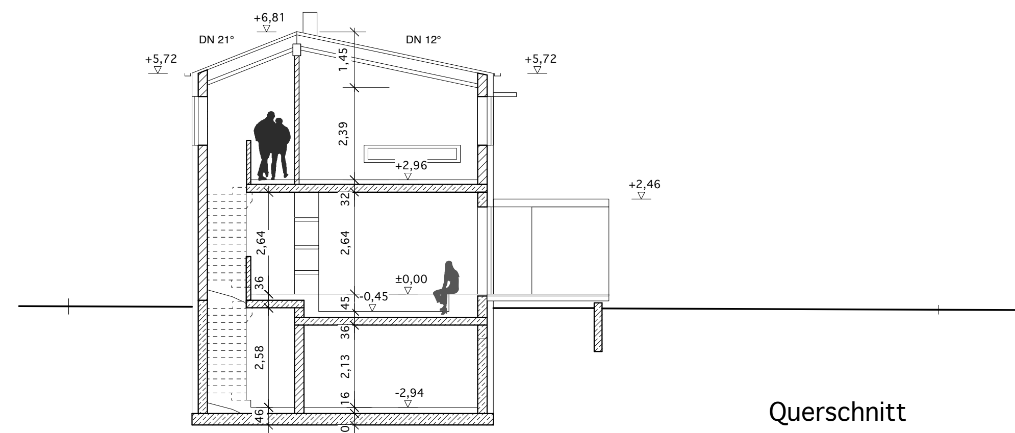
Querschnitt
