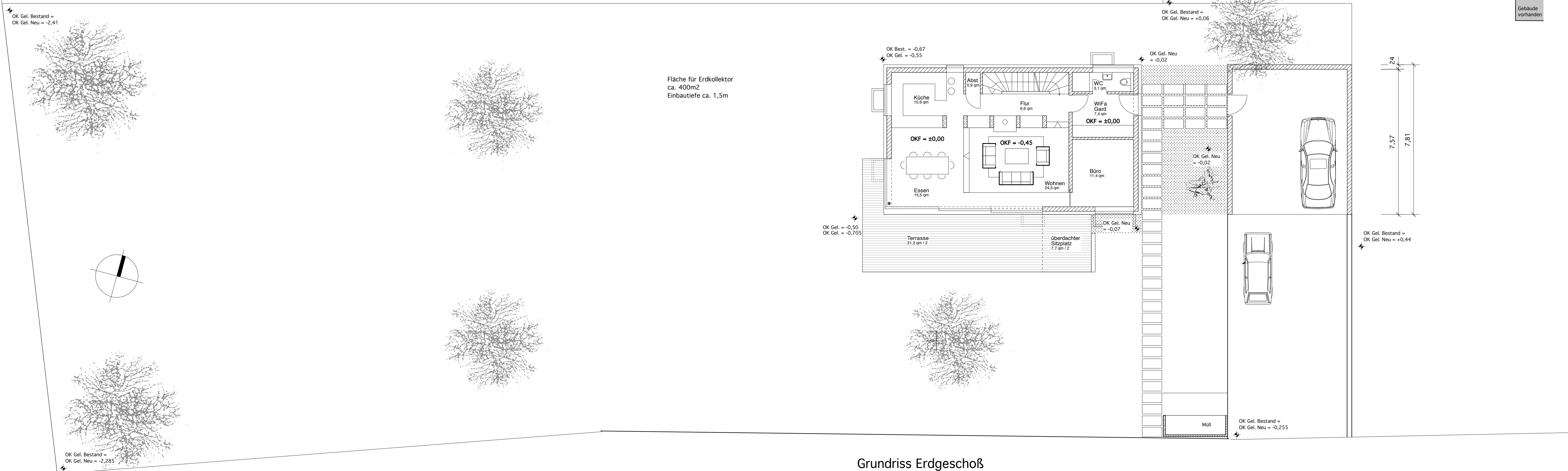
Grundriss Erdgeschoß
