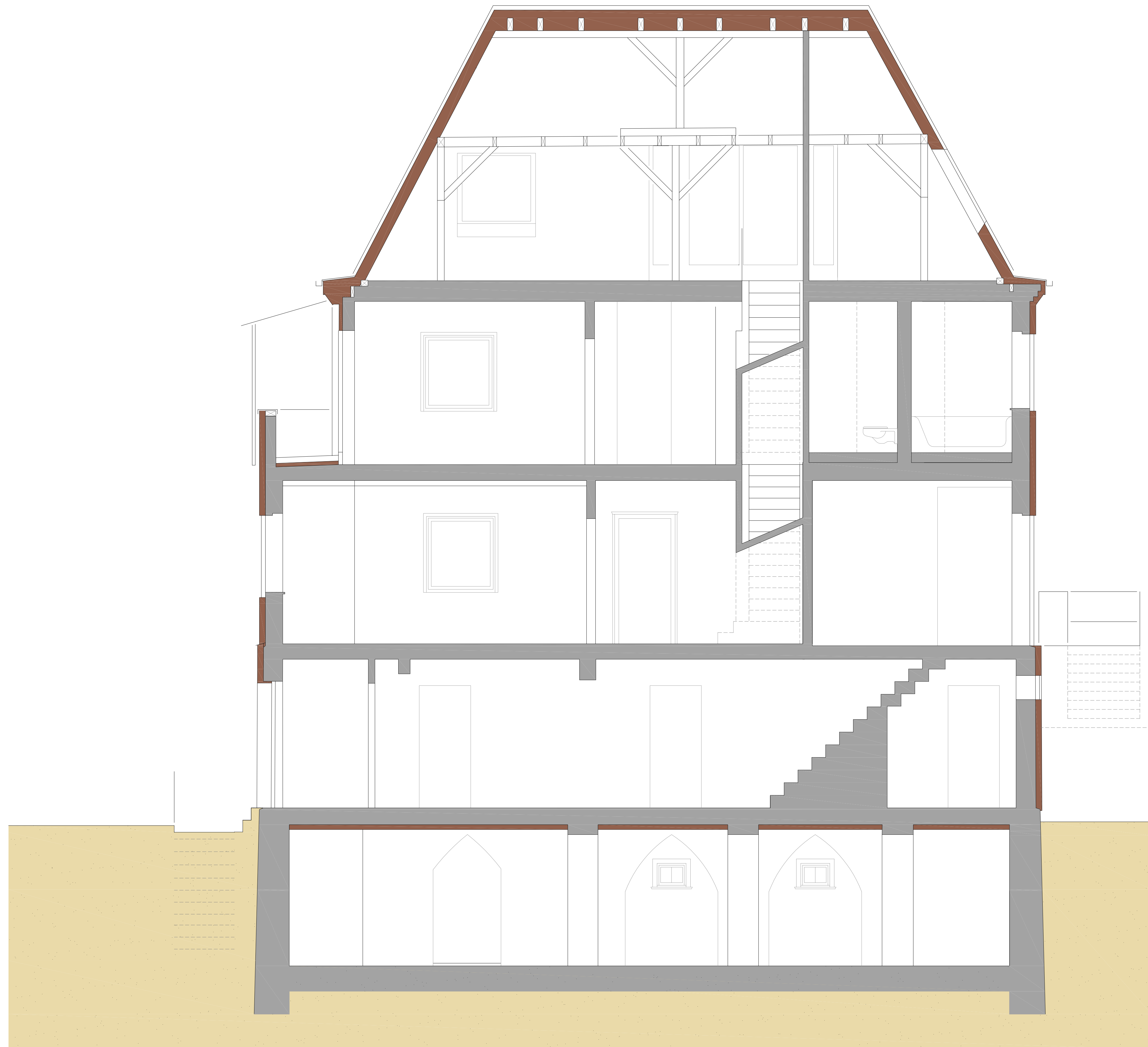
Längsschnitt
