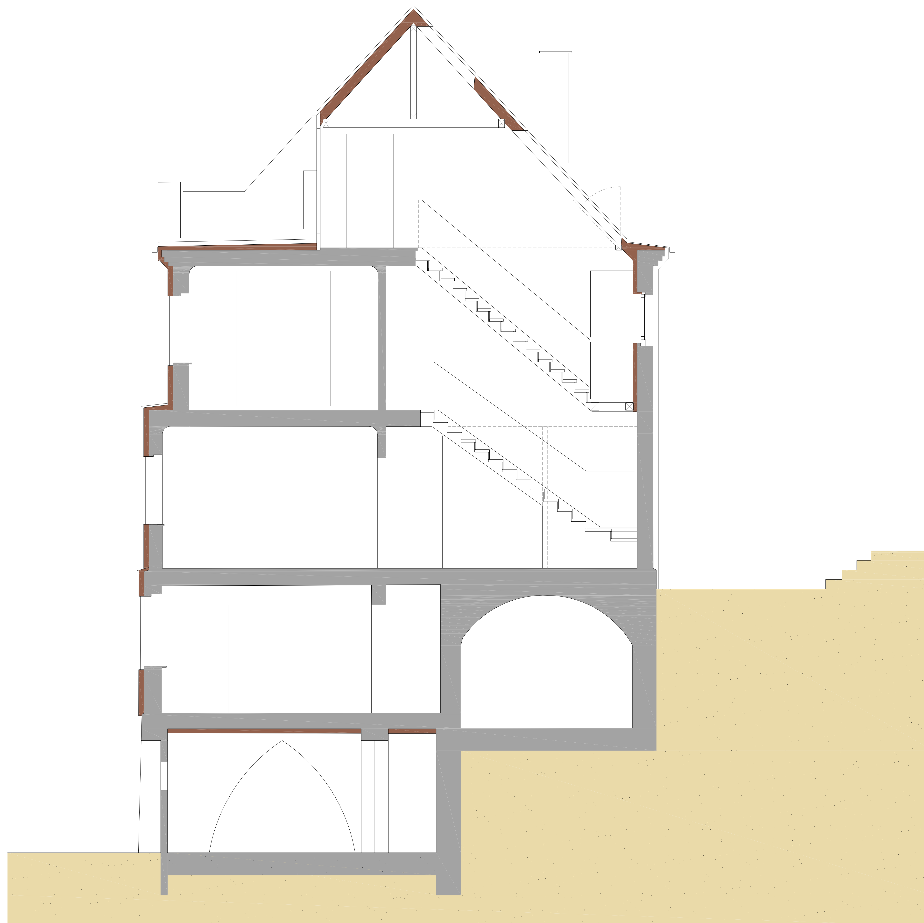
Querschnitt
