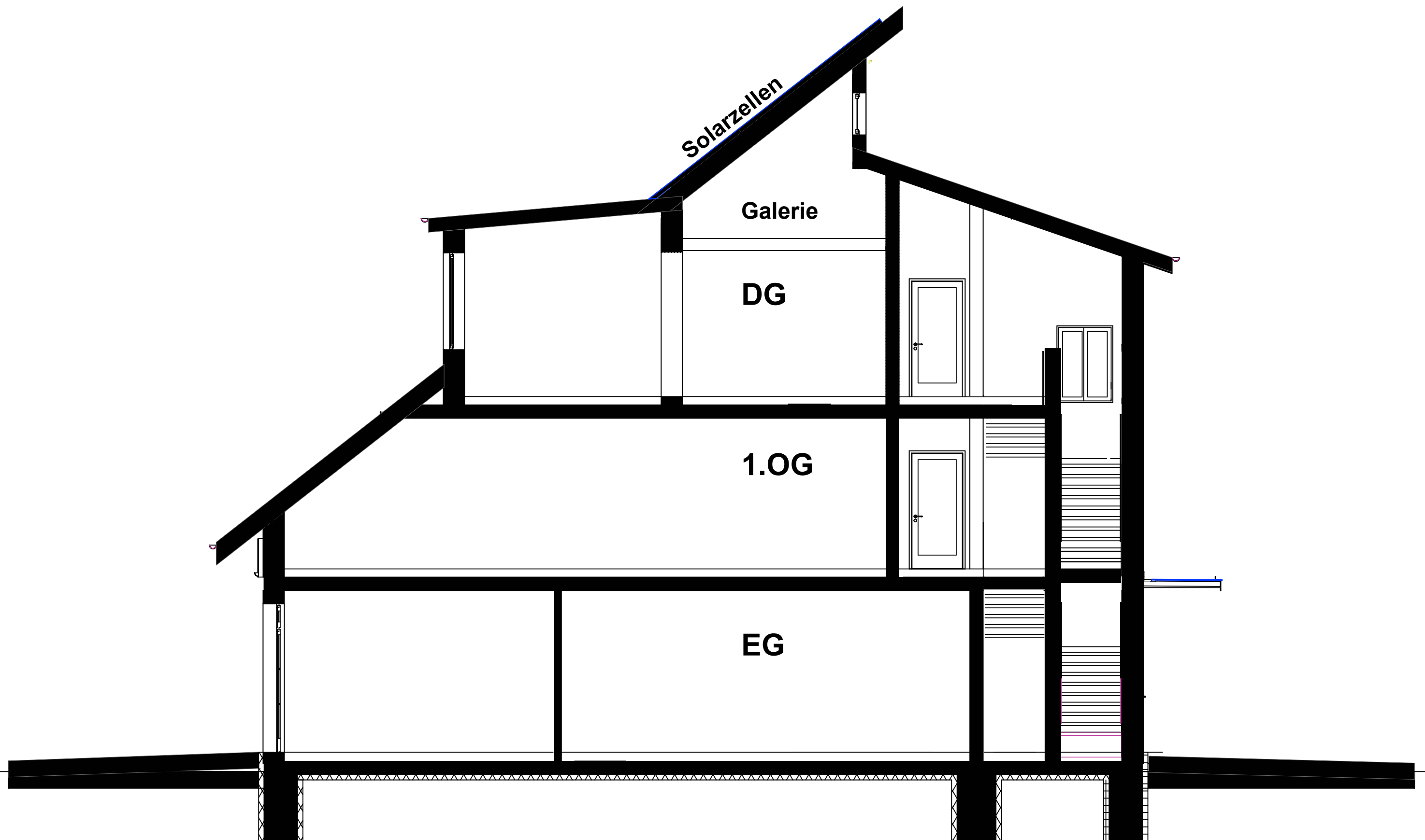
Schnitt
