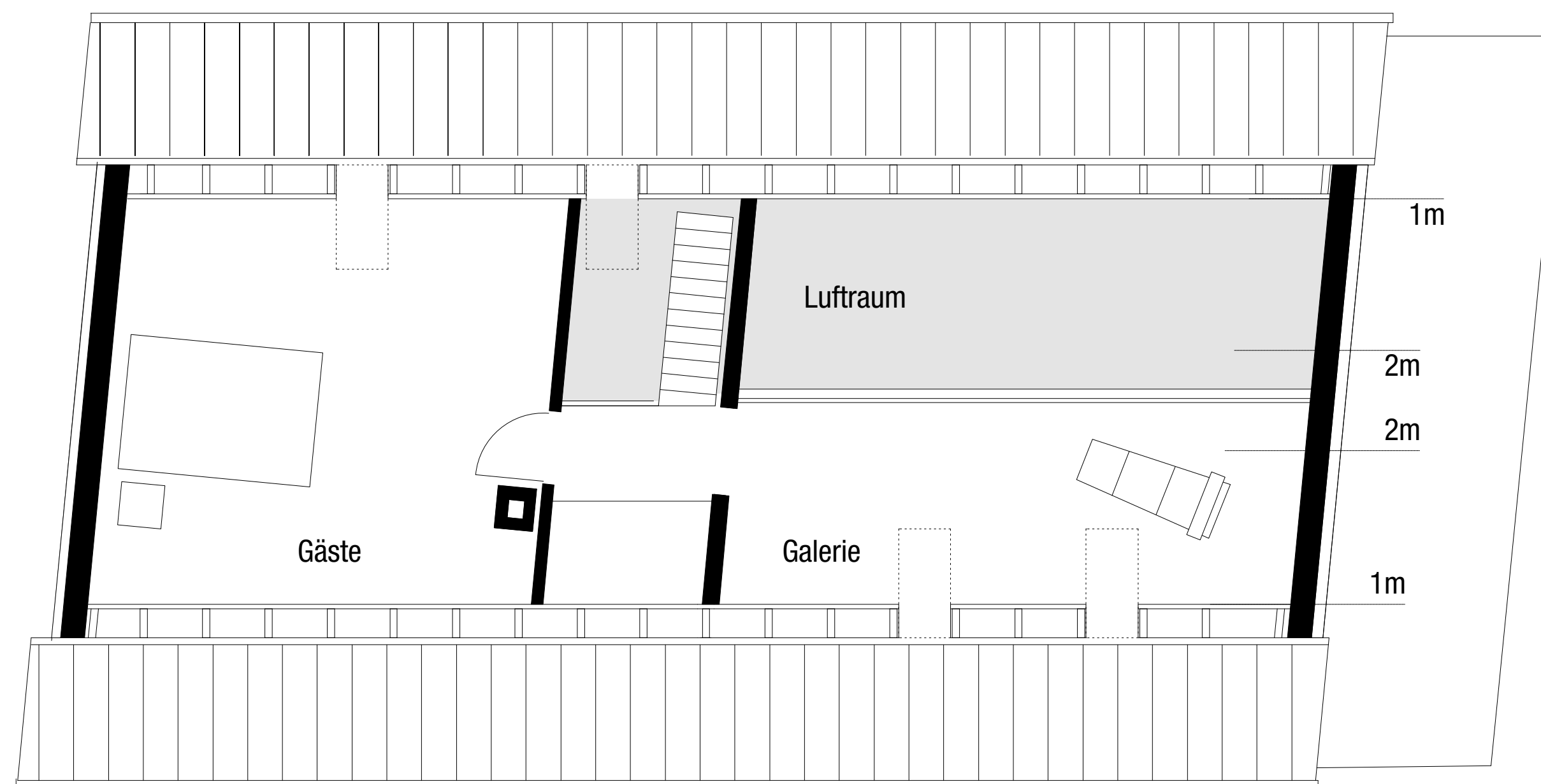
Grundriß Dachgeschoß
