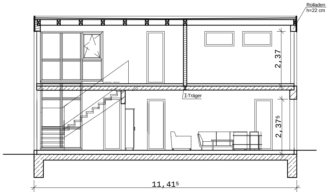
Schnitt
