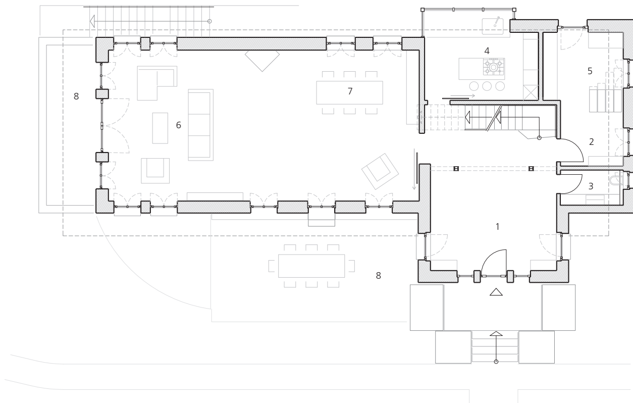
Haus S Grundriss Erdgeschoss
