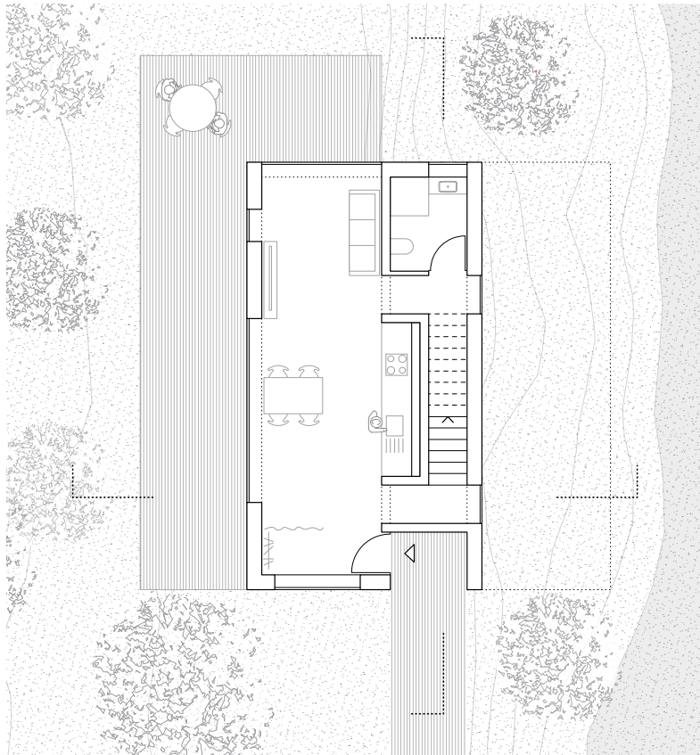
Grundriss Erdgeschoss
