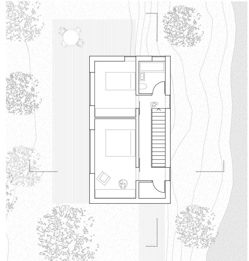
Grundriss Obergeschoss
