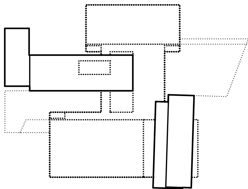
Bestand / Neubau
