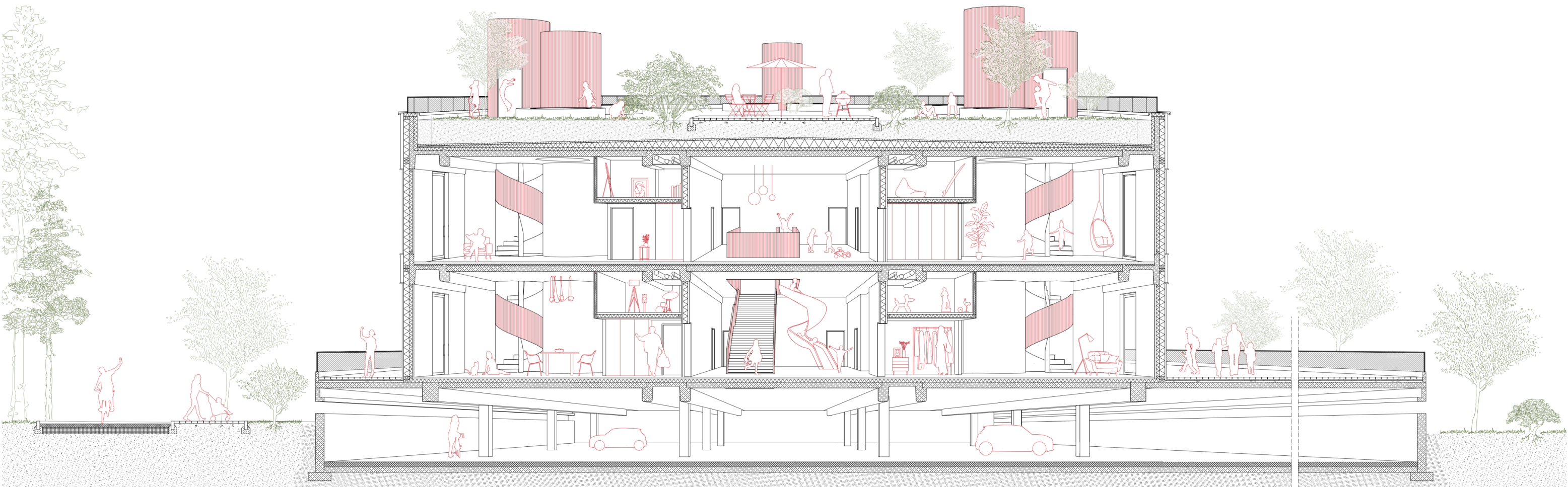
Schnittperspektive 1:50
