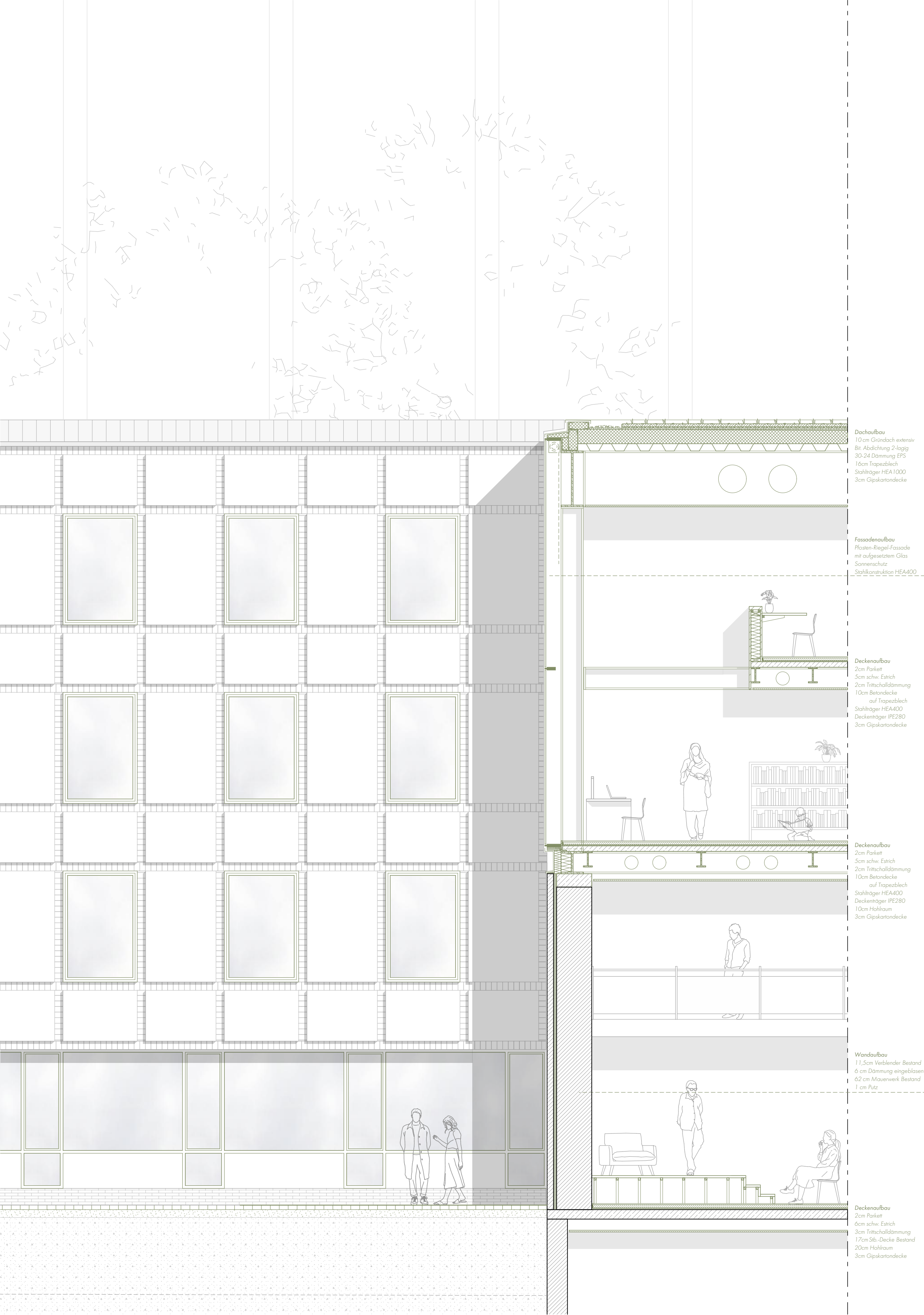
Fassadenschnitt Aufstockung Bibliothek 1.50
