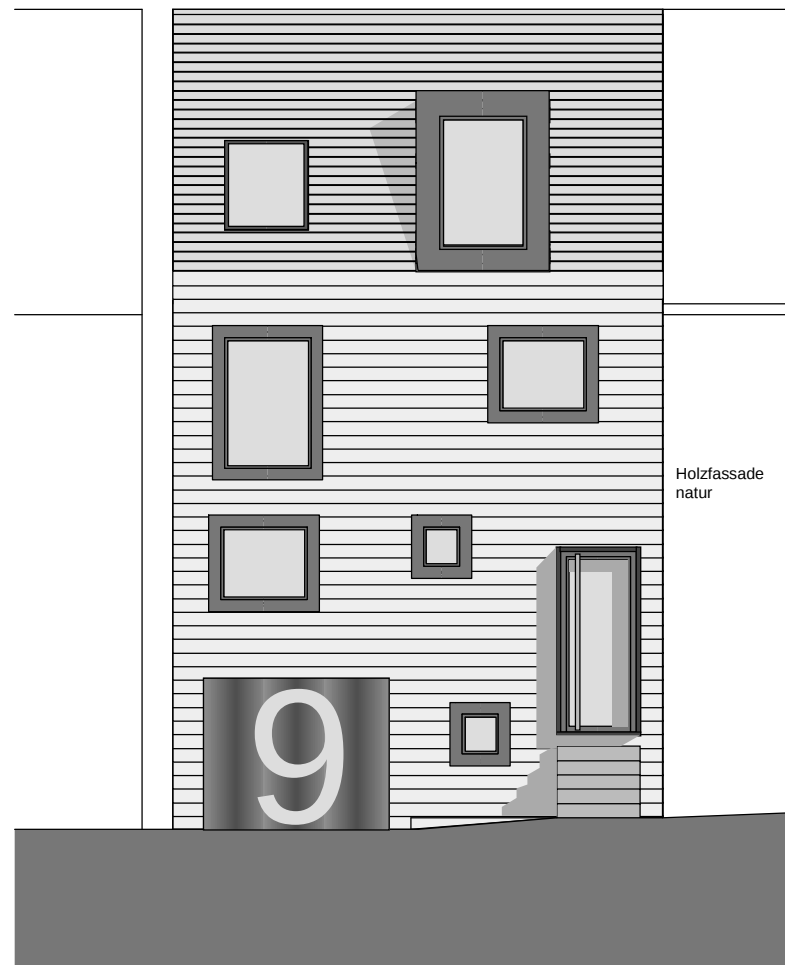
Ostansicht
