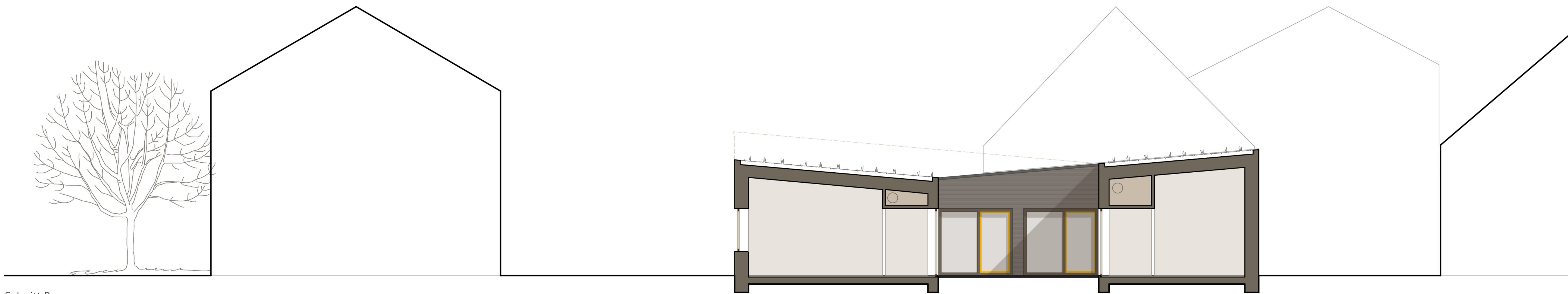
Schnitt B
