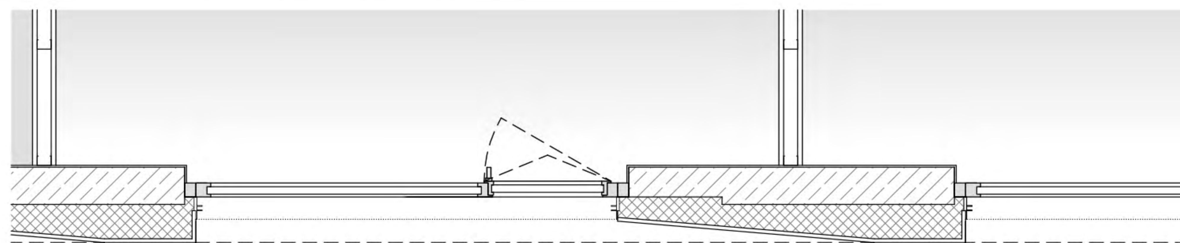
FASSADENSCHNITT M 1:50
