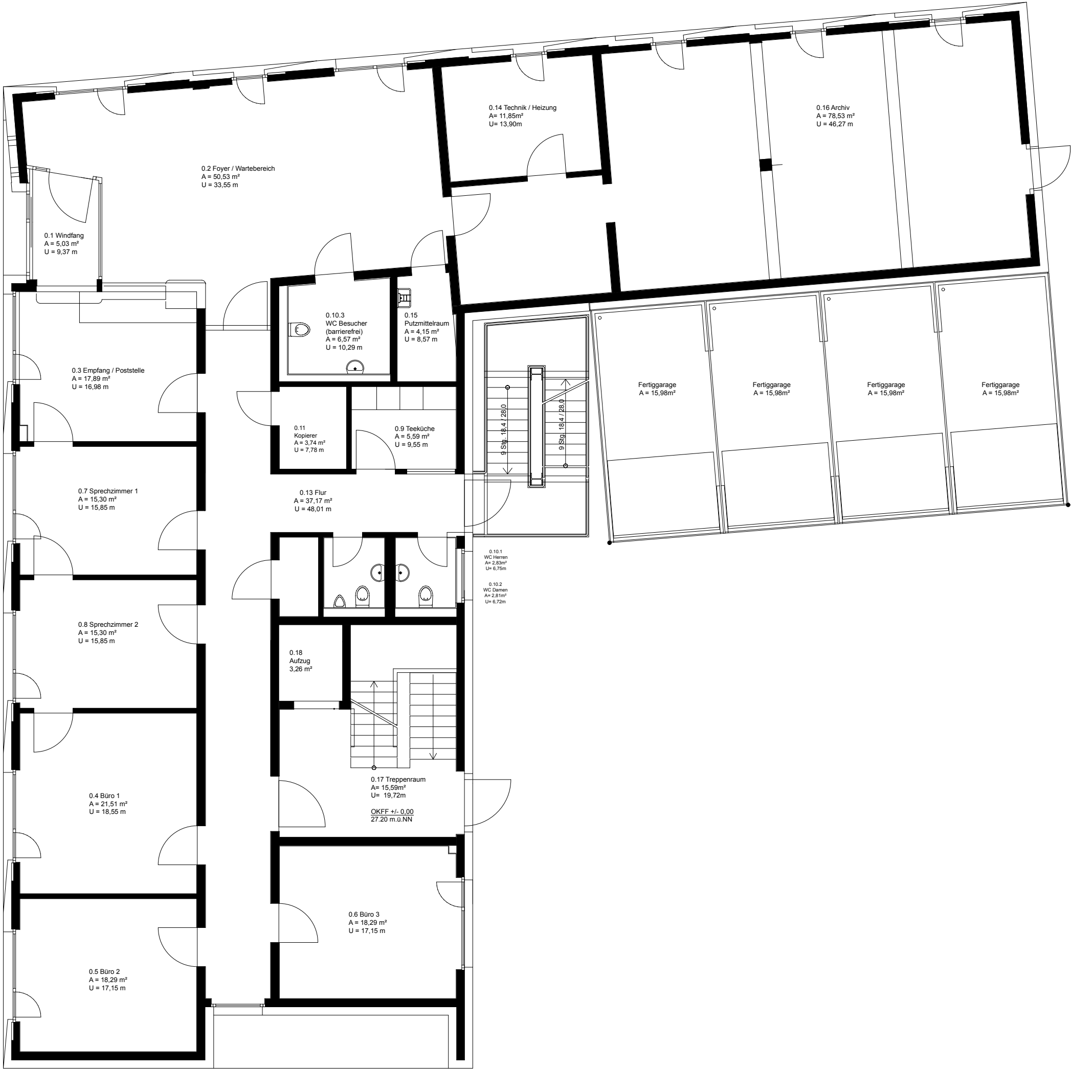
Grundriss Erdgeschoss
