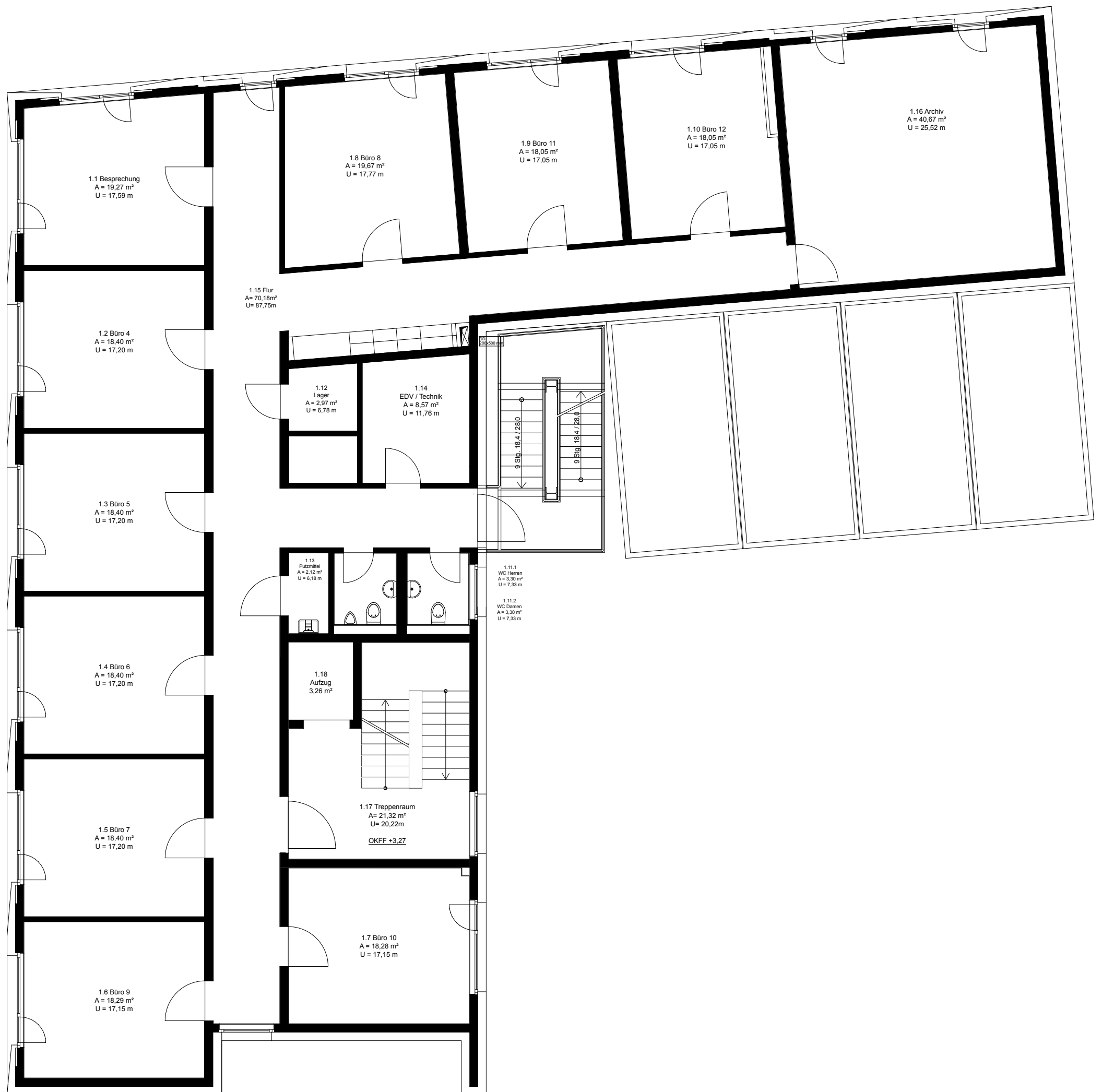
Grundriss 1. Obergeschoss
