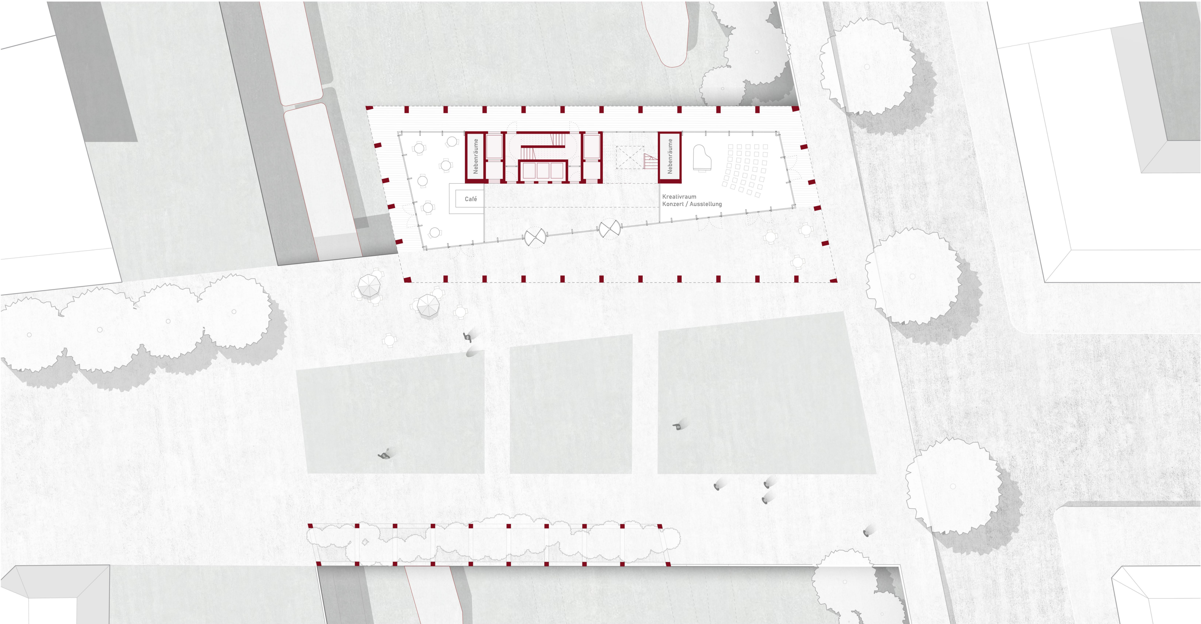
GRUNDRISS EG M 1:200
