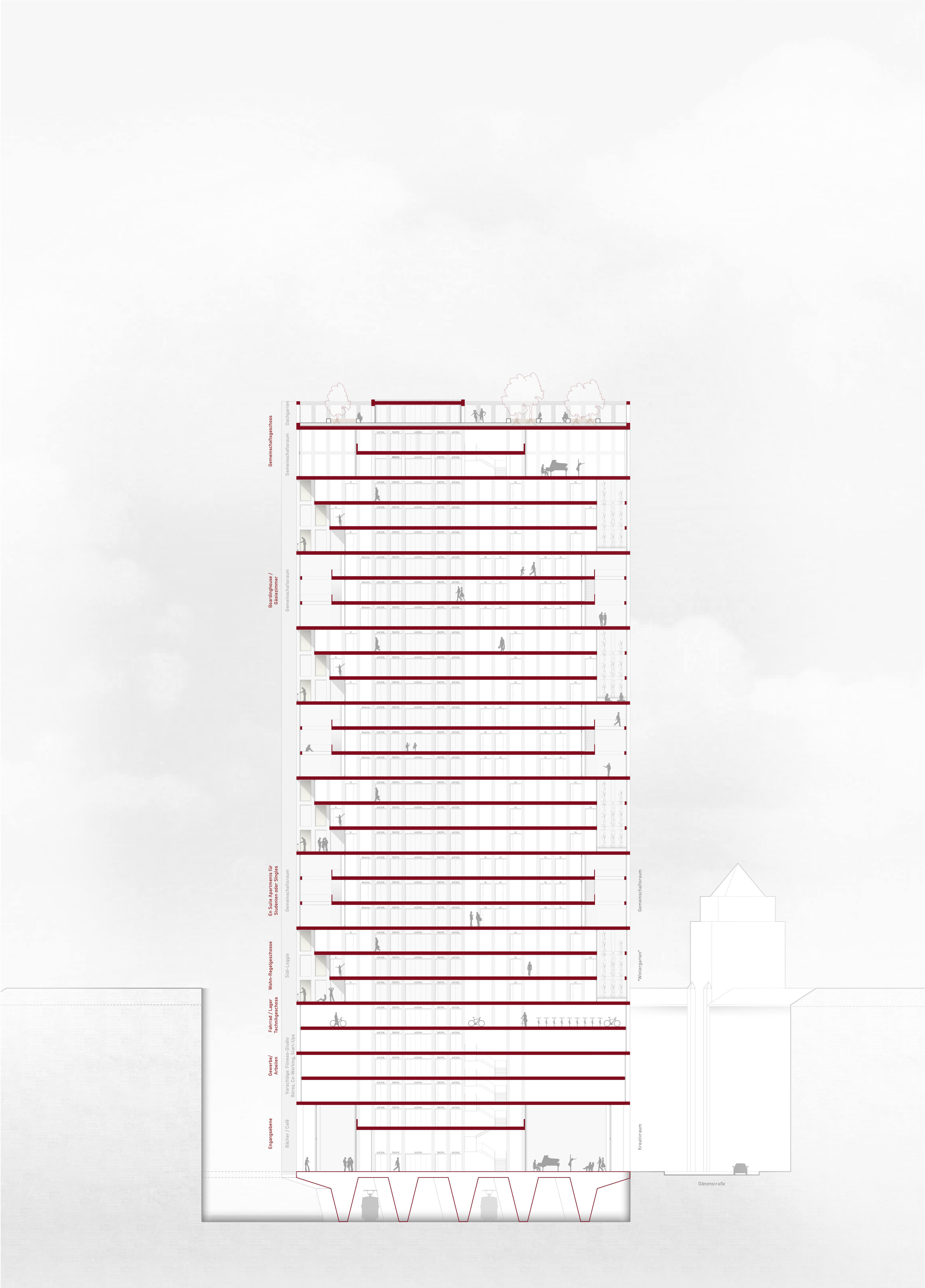
SCHNITT M 1:200
