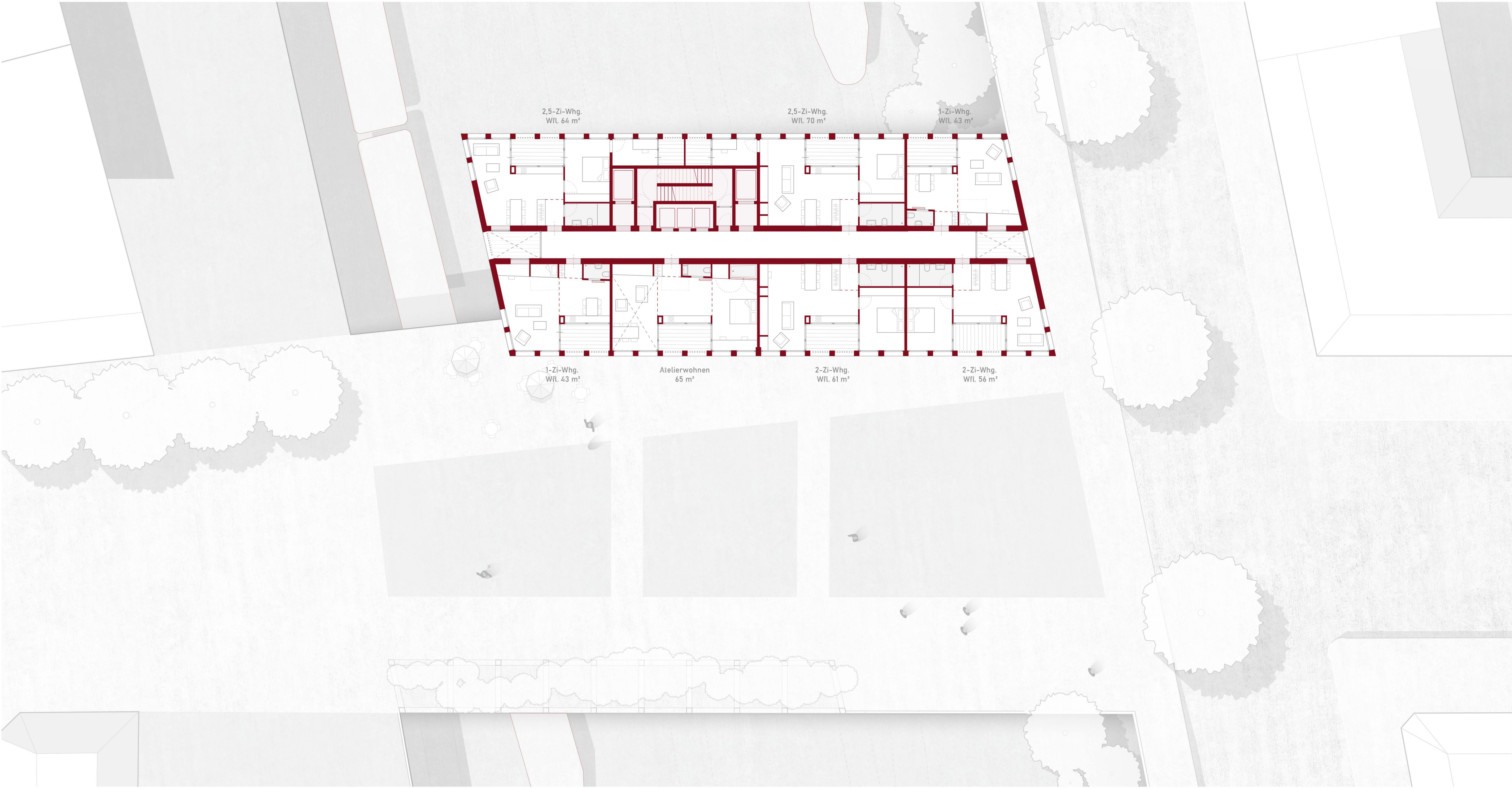
IG GRUNDRISS WOHNREGELGESCHOSS M 1:20
