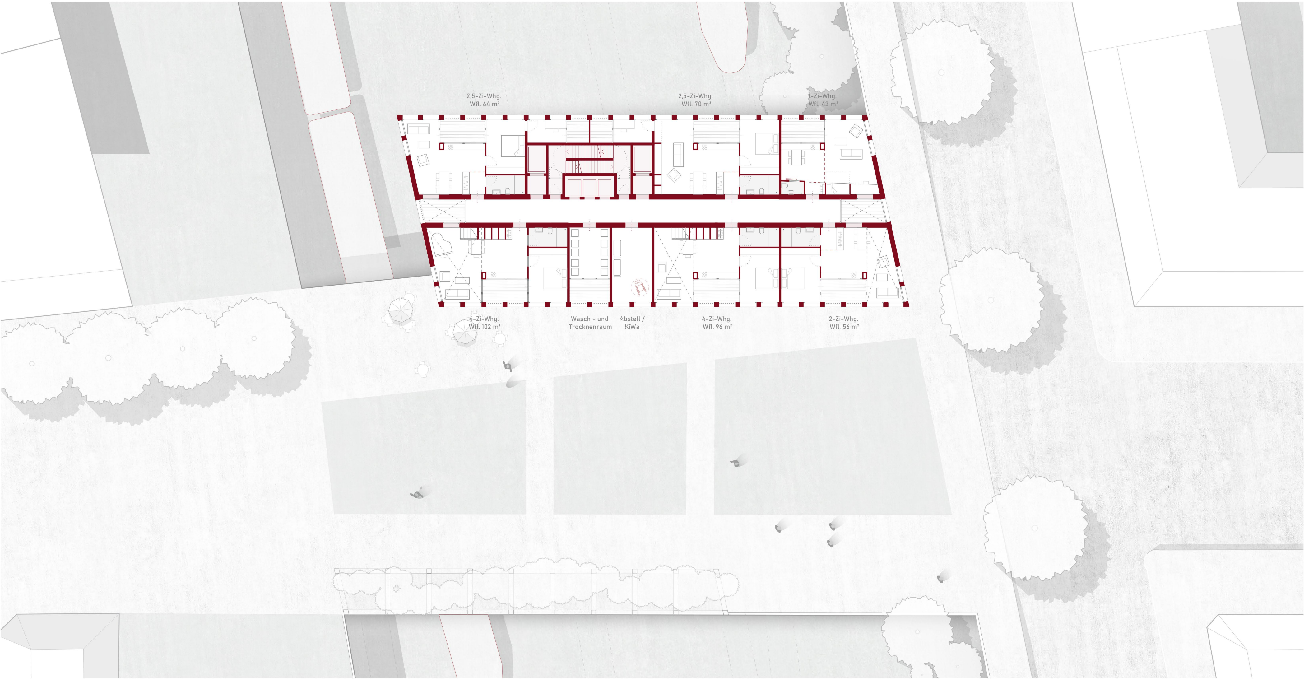
IG GRUNDRISS WOHNEN MAISONETTE 1 M 1:20
