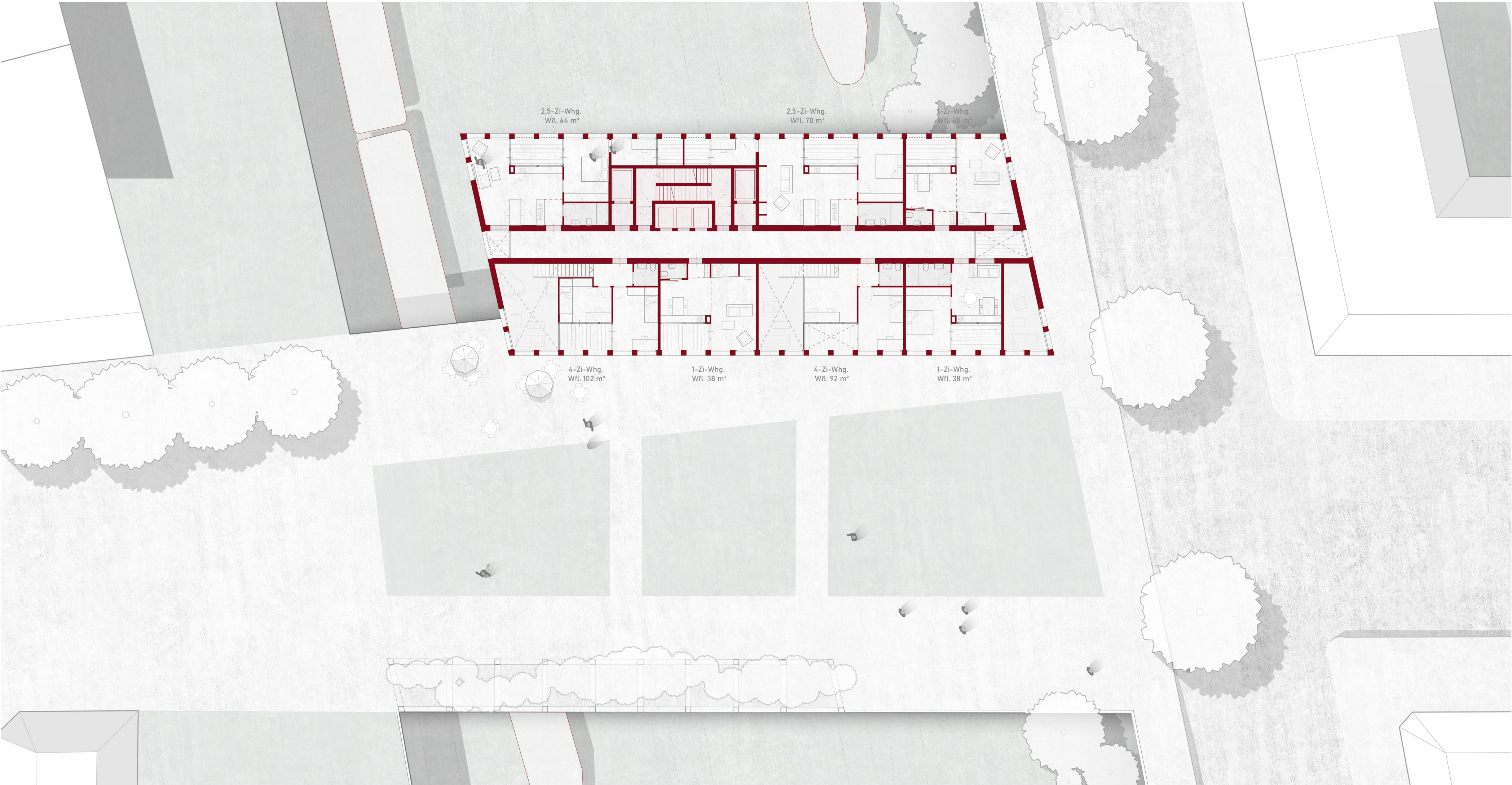
OG GRUNDRISS WOHNEN MAISONETTE 2 M 1:
