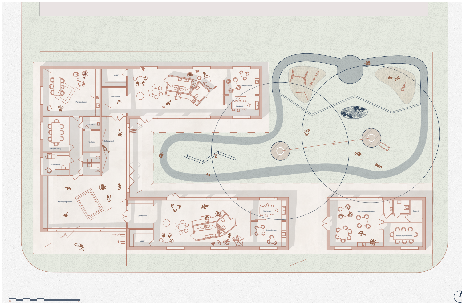
GRUNDRISS
