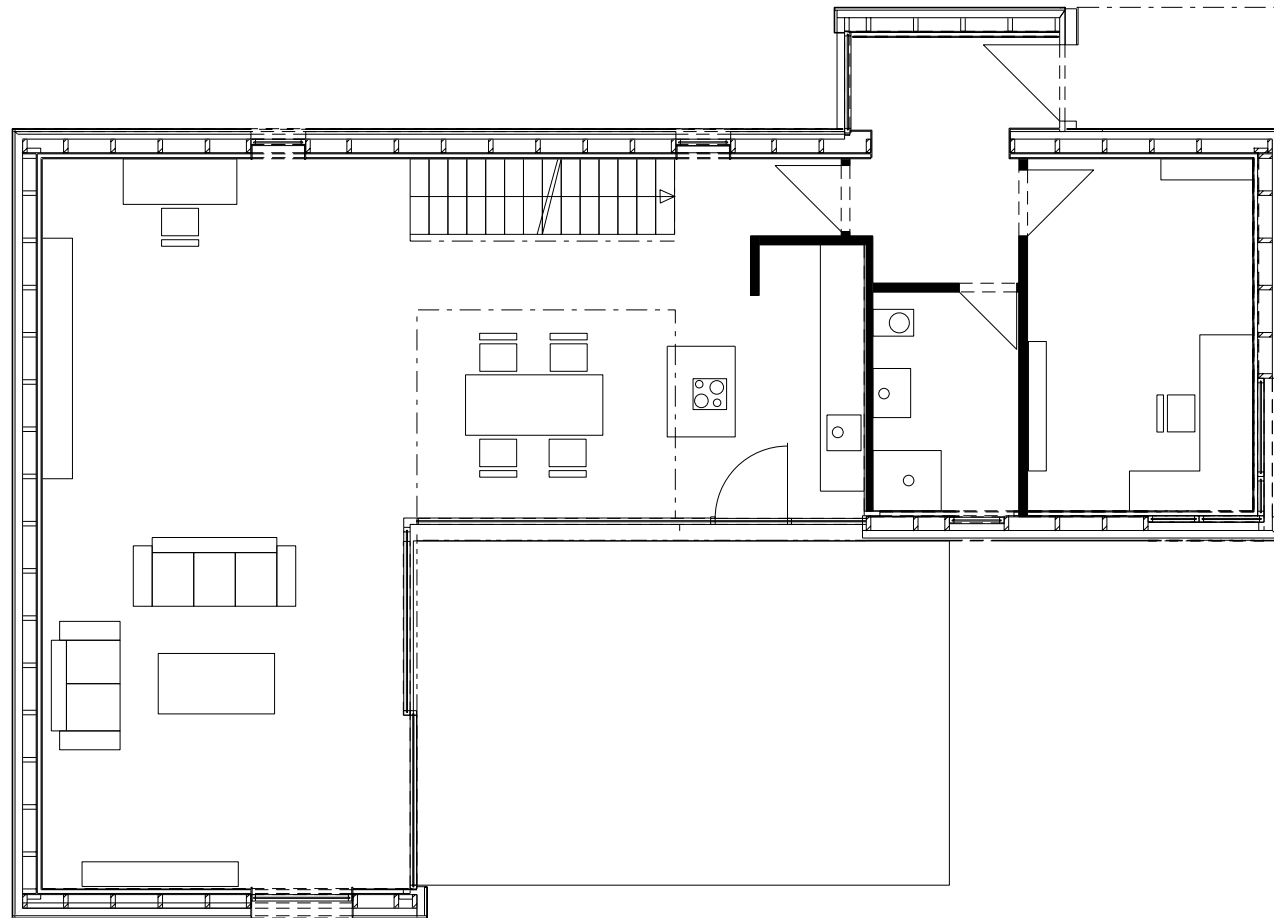
Grundriss EG
