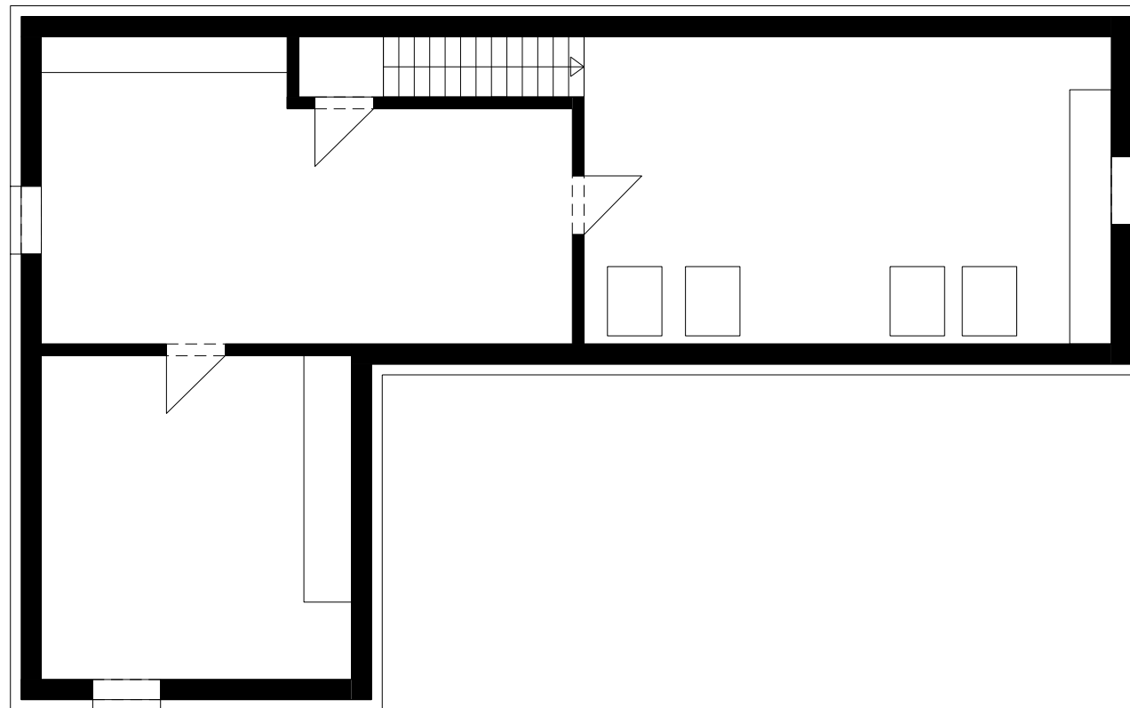
Grundriss KG
