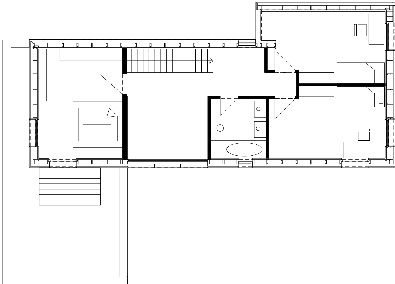
Grundriss OG
