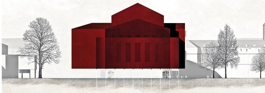
Ansicht Nord | M1:200
