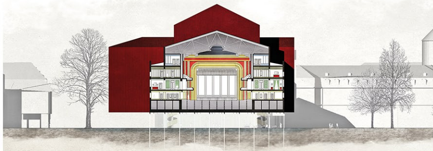
Querschnitt | M1:200
