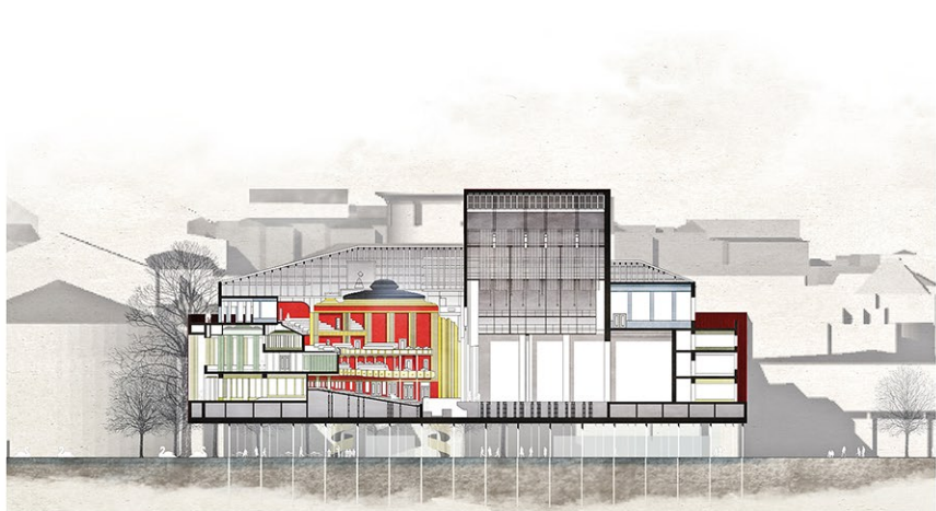
Längsschnitt | M1:200
