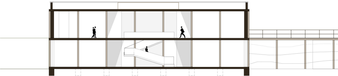
Schnitt I-I
