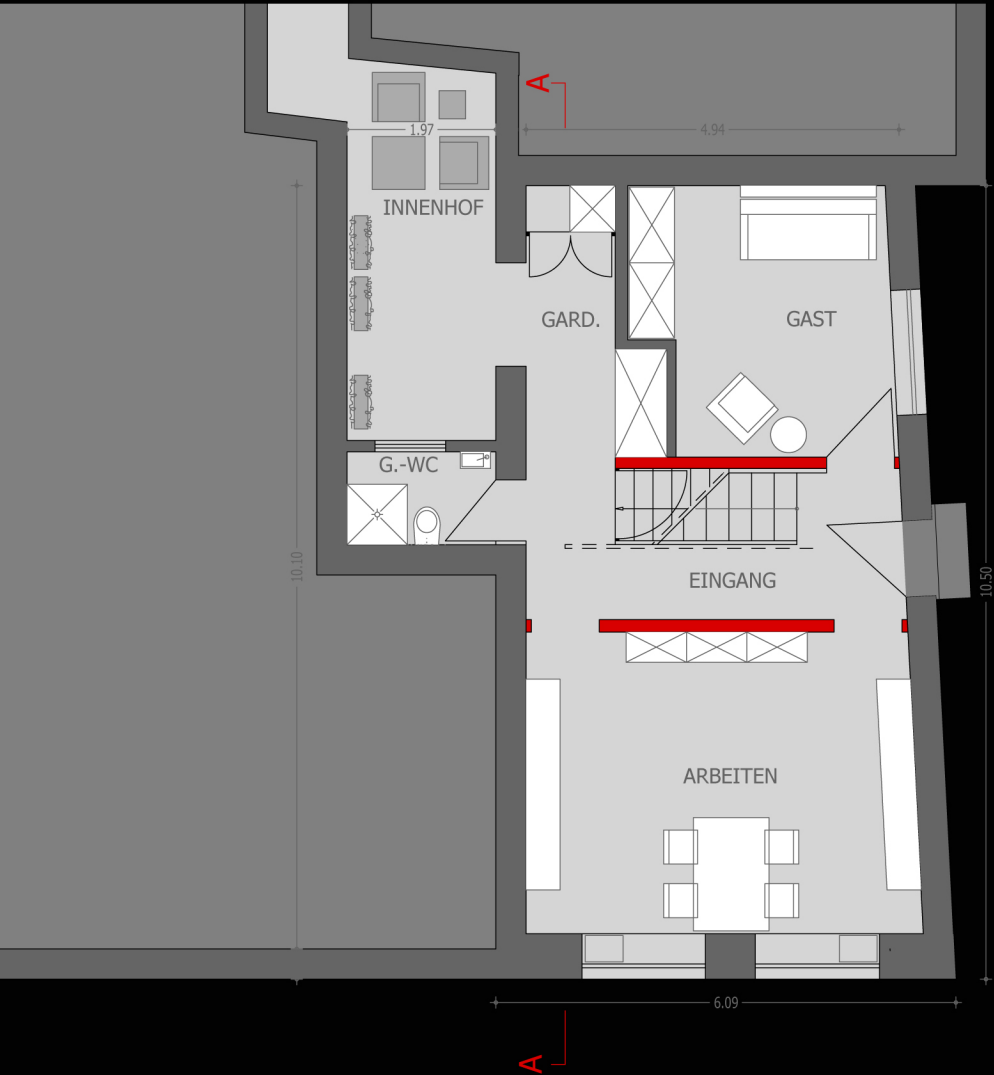
Grundriss Erdgeschoss 1:100
