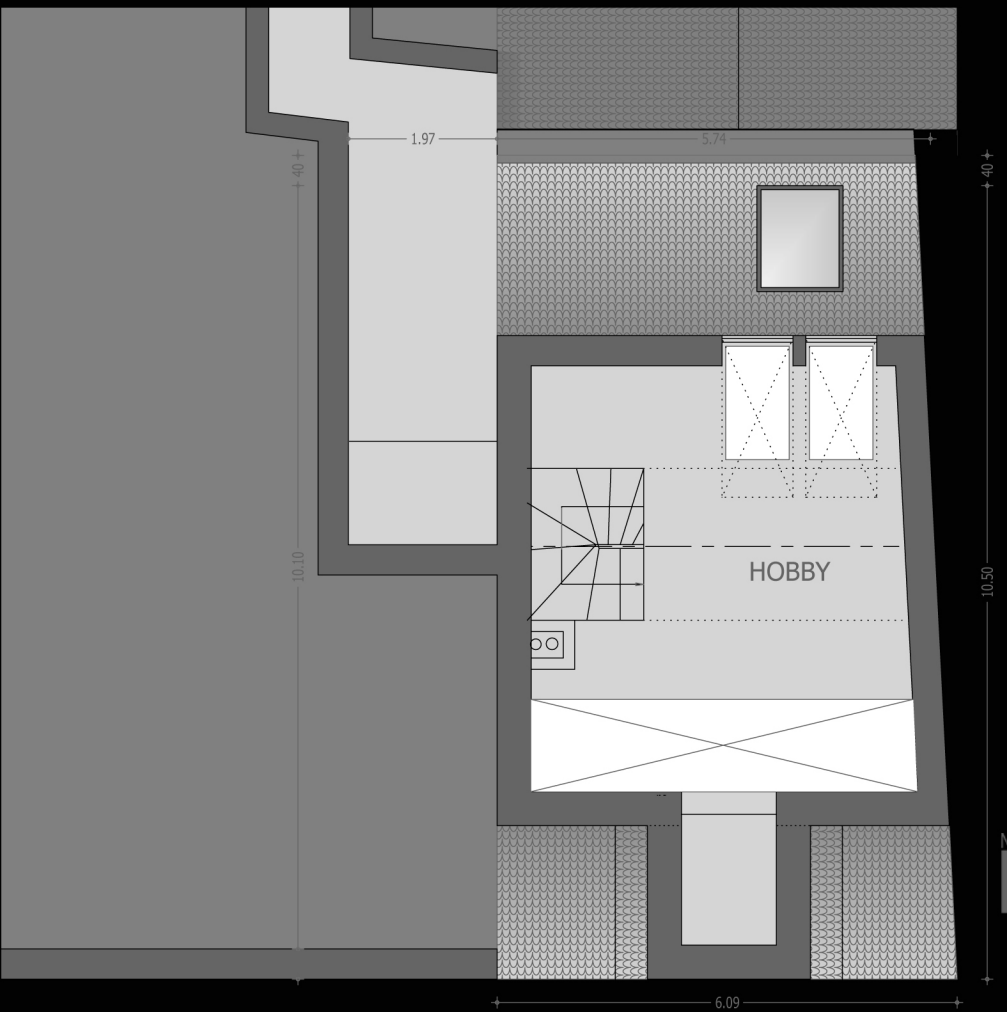
Grundriss Dachgeschoss 1:100
