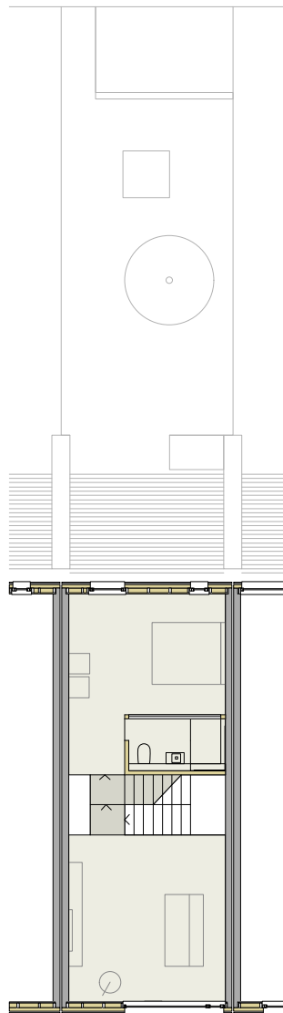
1.OG
