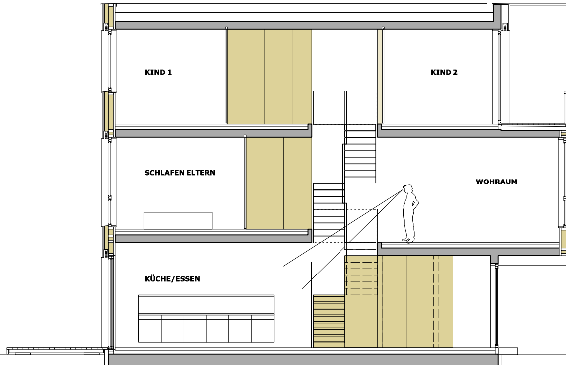
SCHNITT
