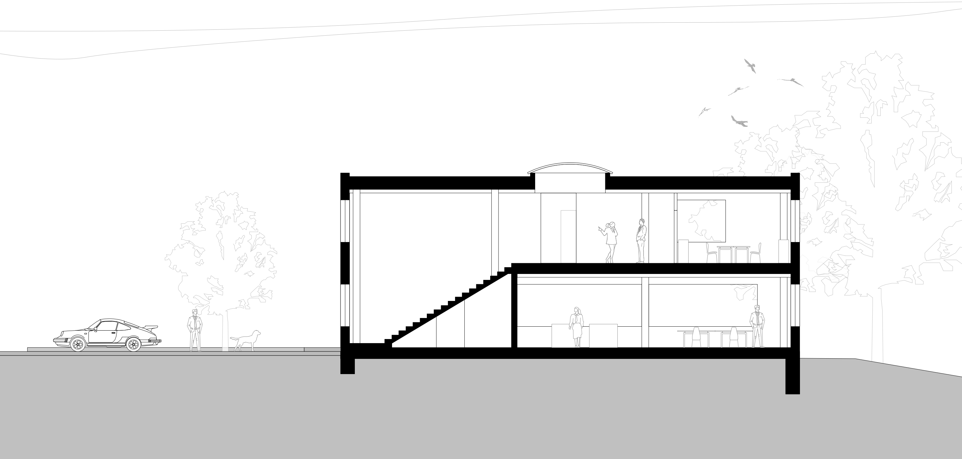
Schnitt A-A M 1:100
