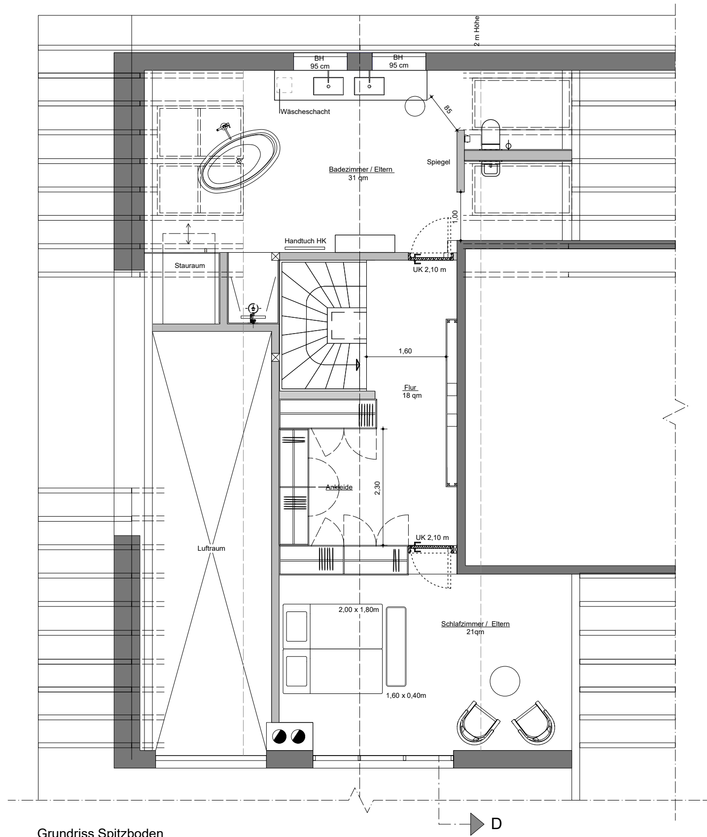
Grundriss Spitzboden
