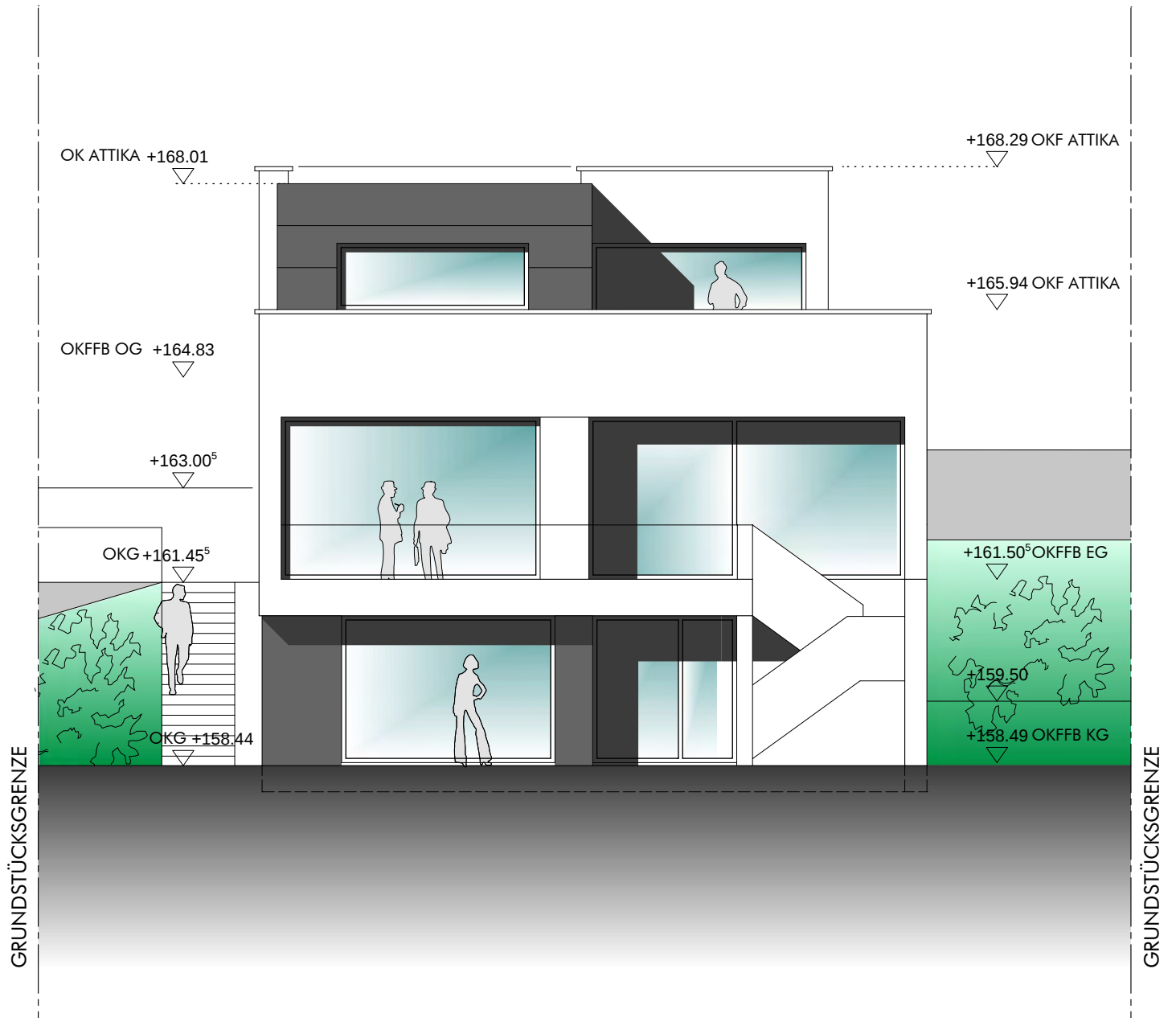
ANSICHT GARTEN
