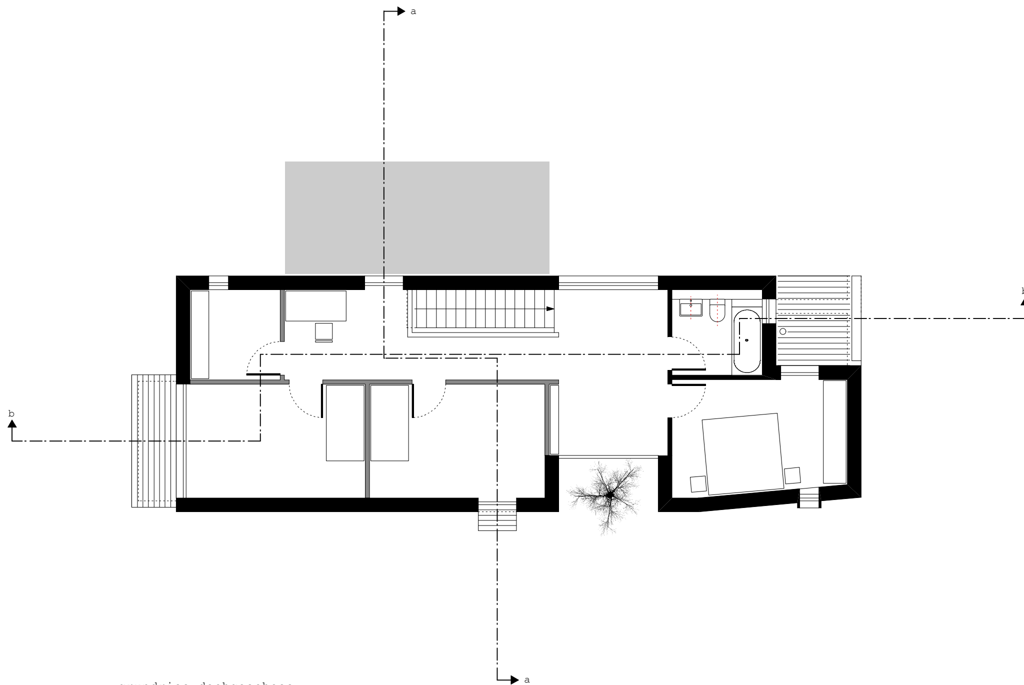
grundriss dachgeschoss
