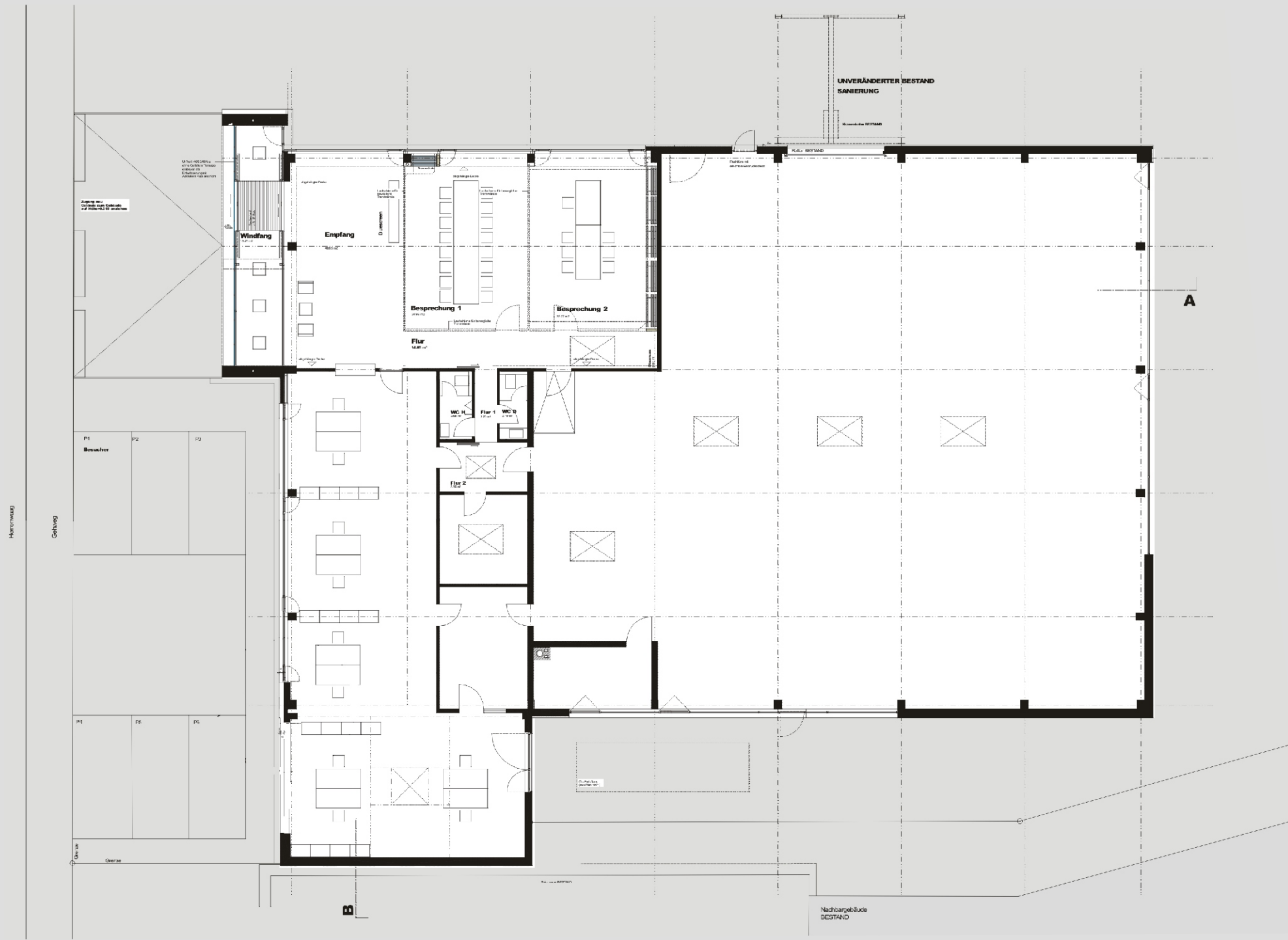
grundriss
