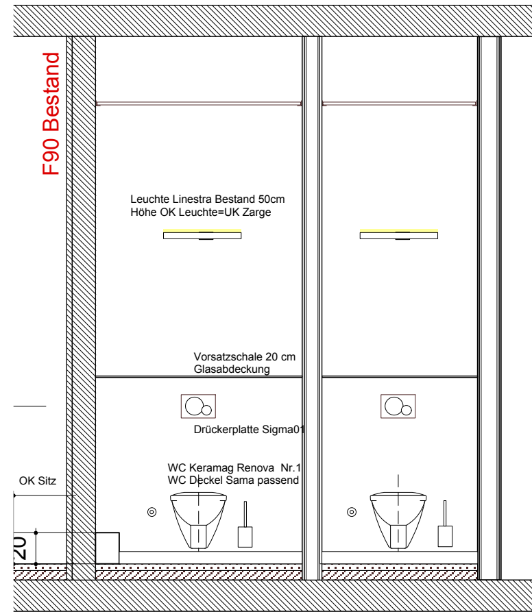
SNITT B-B'
