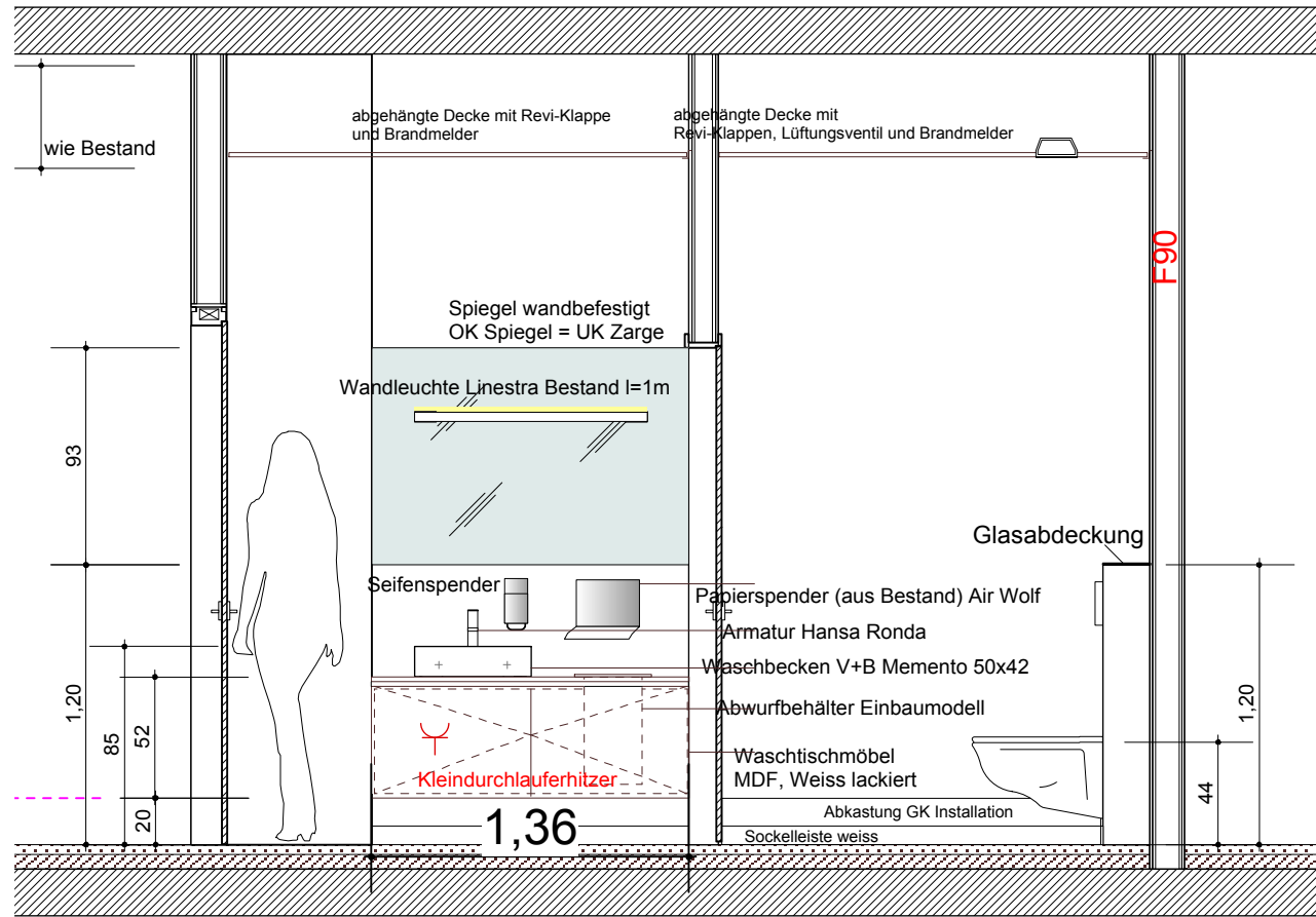
SNITT A-A'
