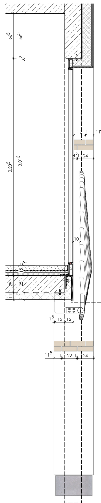
Detailschnitt
