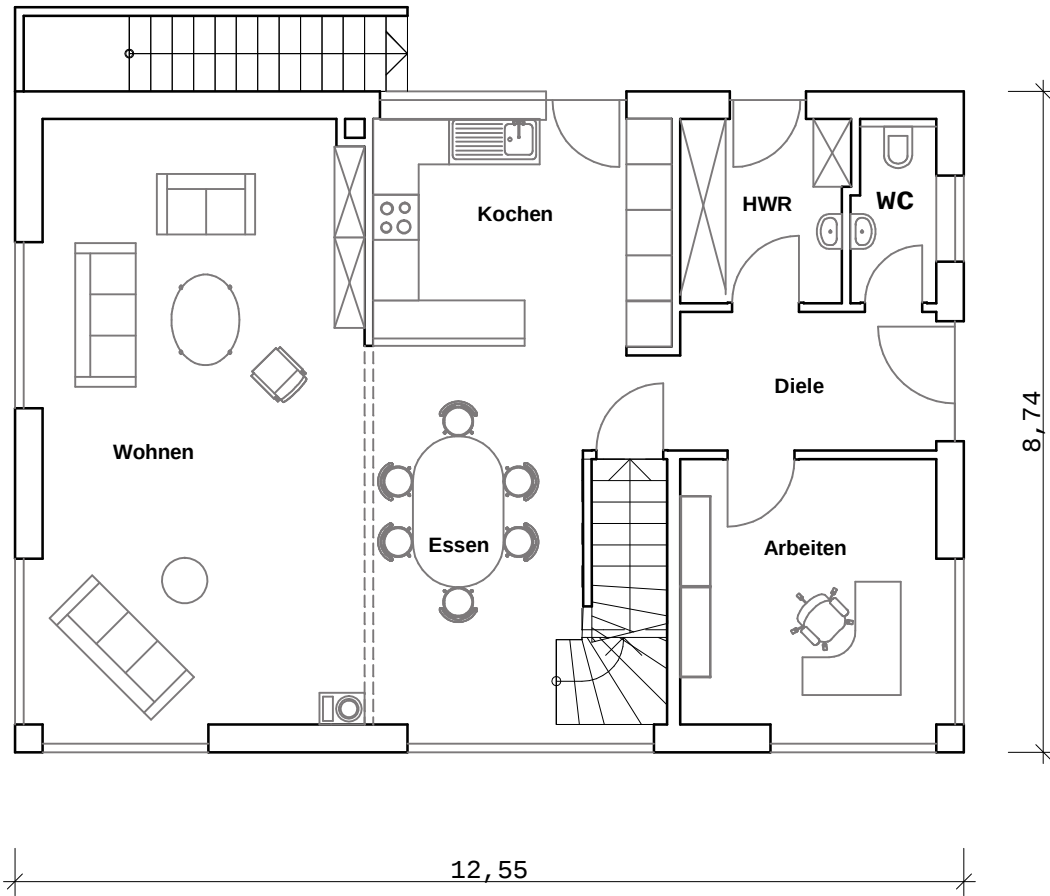
Grundriss Erdgeschoss
