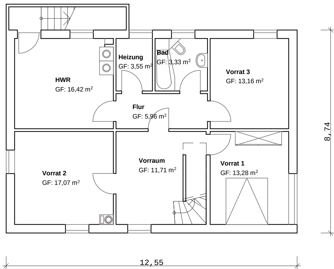
Grundriss Kellergeschoss
