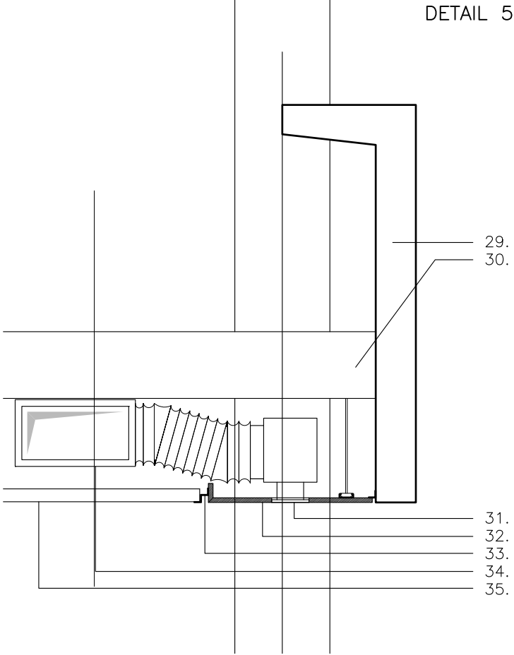
LEGENDE DETAILS 4 ET 5 – OUVRANT DE CONFORT ET CIRCULATION EN MEZZANINE
