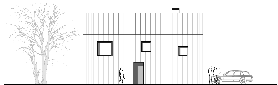
Ansicht Ost
