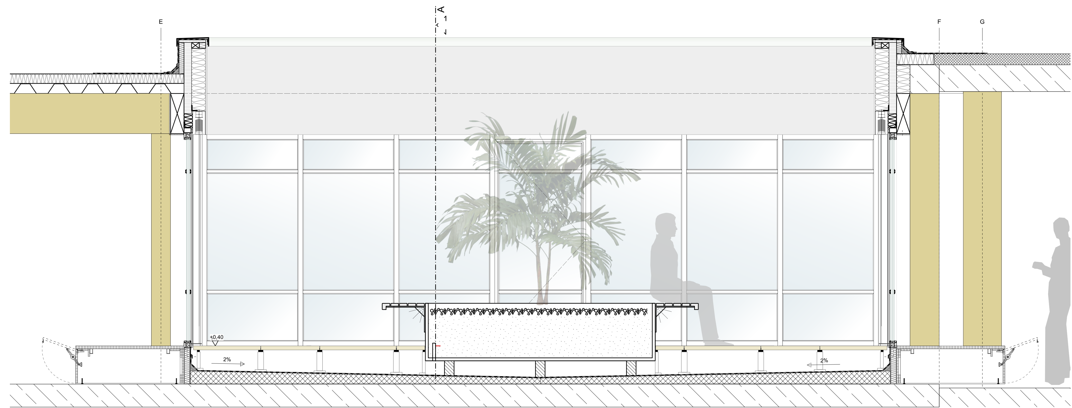
Schnitt B-B M 1:20
