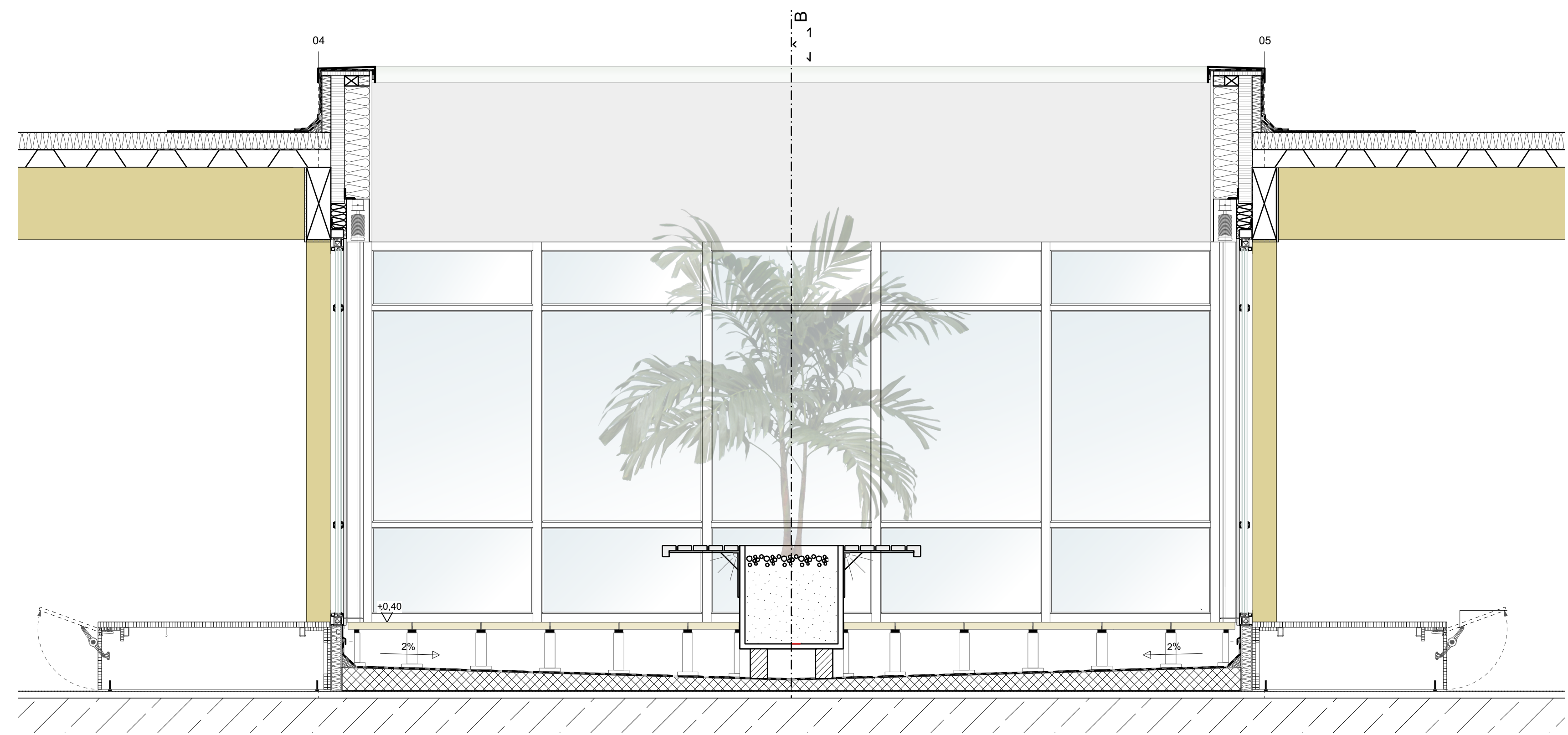
Schnitt A-A M 1:20
