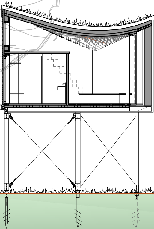
Schnitt A
