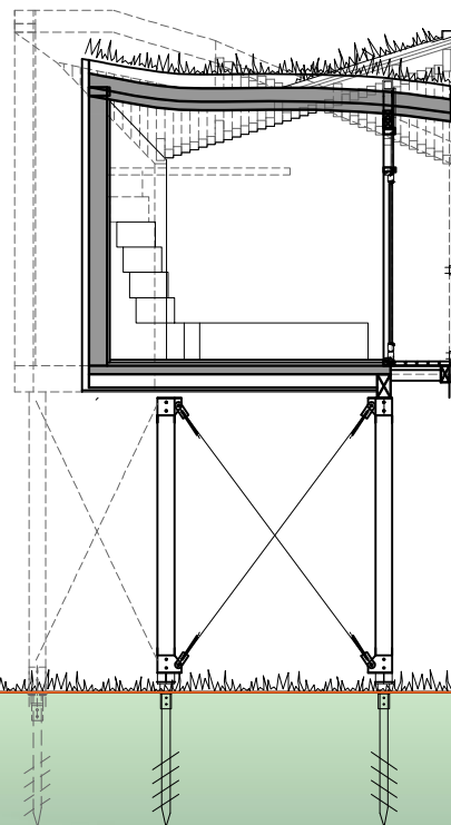
Schnitt C
