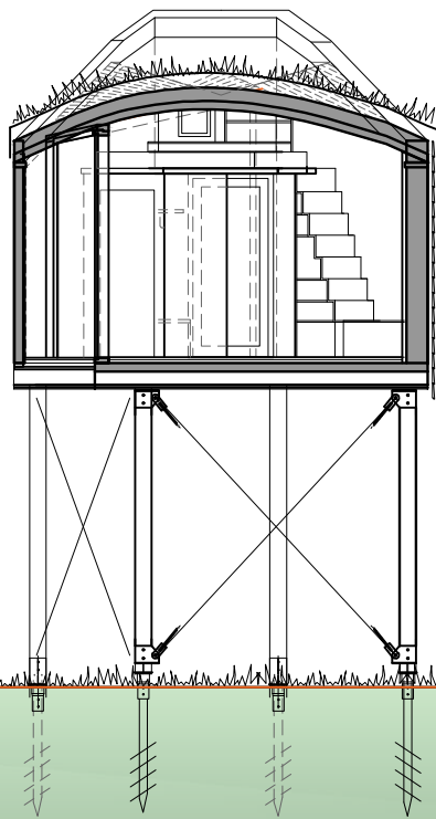
Schnitt B
