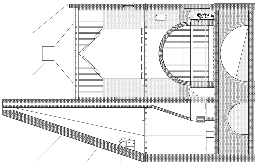
Schnitt I M 1:200
