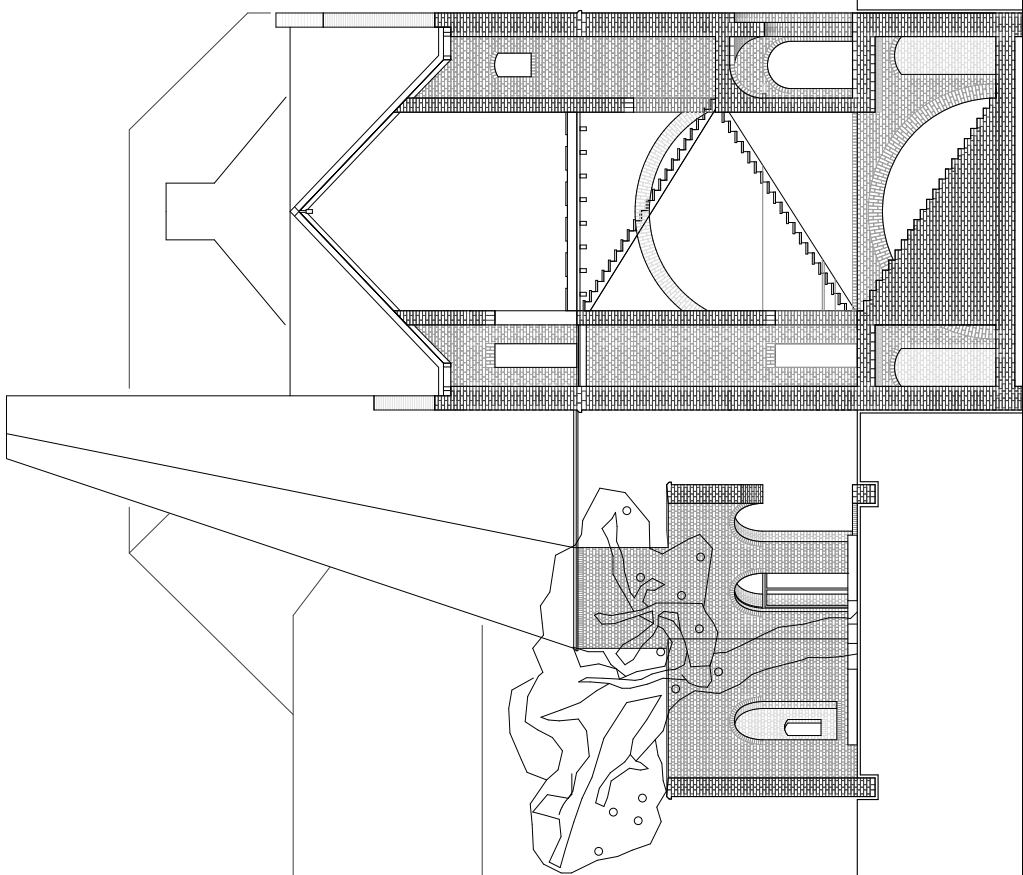
Schnitt II M 1:200
