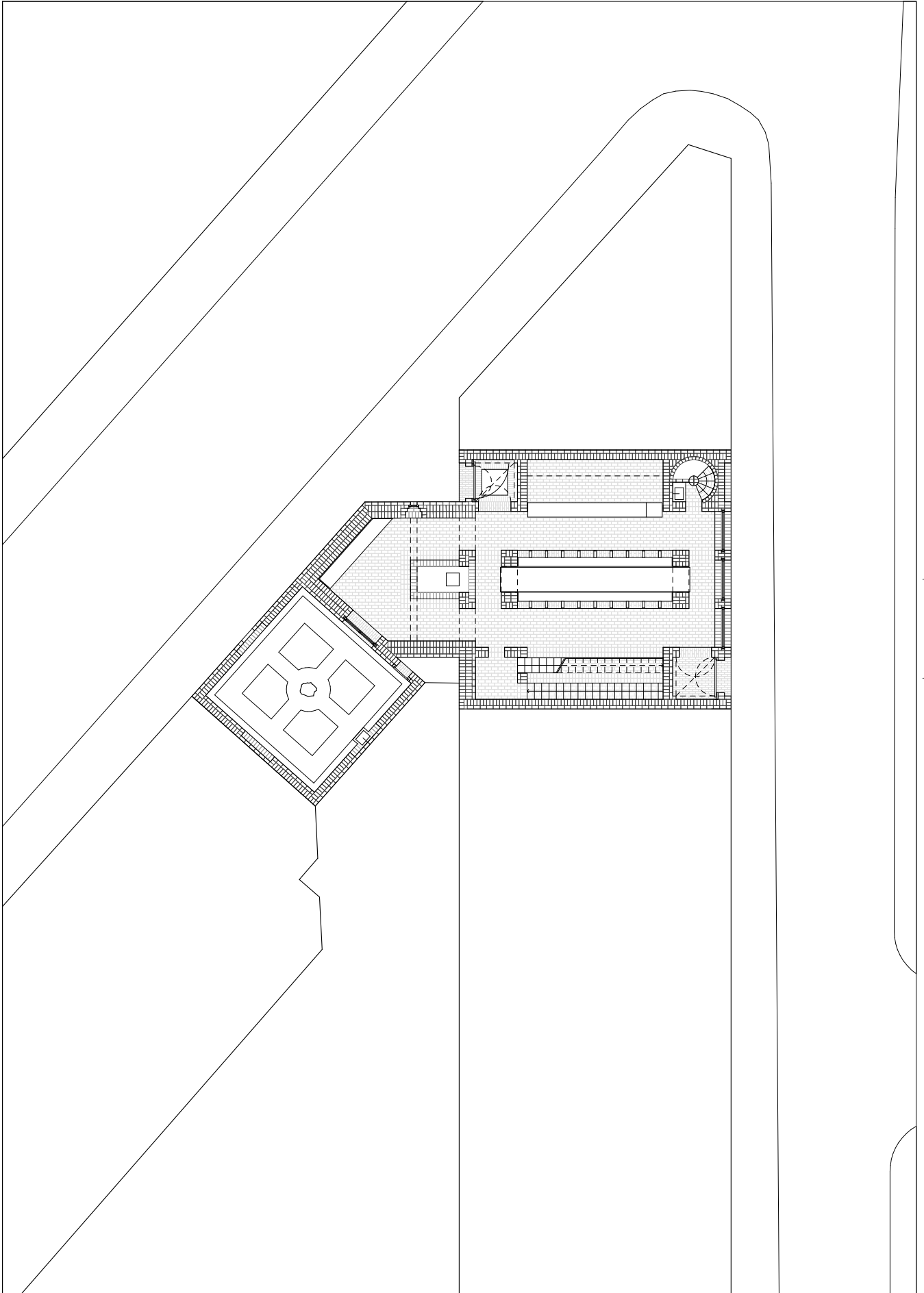
Grundriss 0 M 1:200
